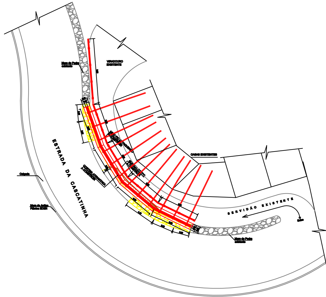
SITUAÇÃO ESCALA 1:250
