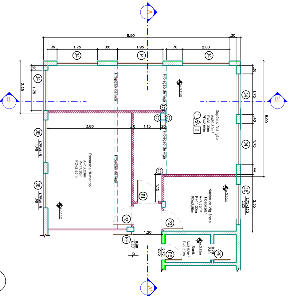
01 PLANTA BAIXA - PAVIMENTO TÉRREO ESC. 1/100
