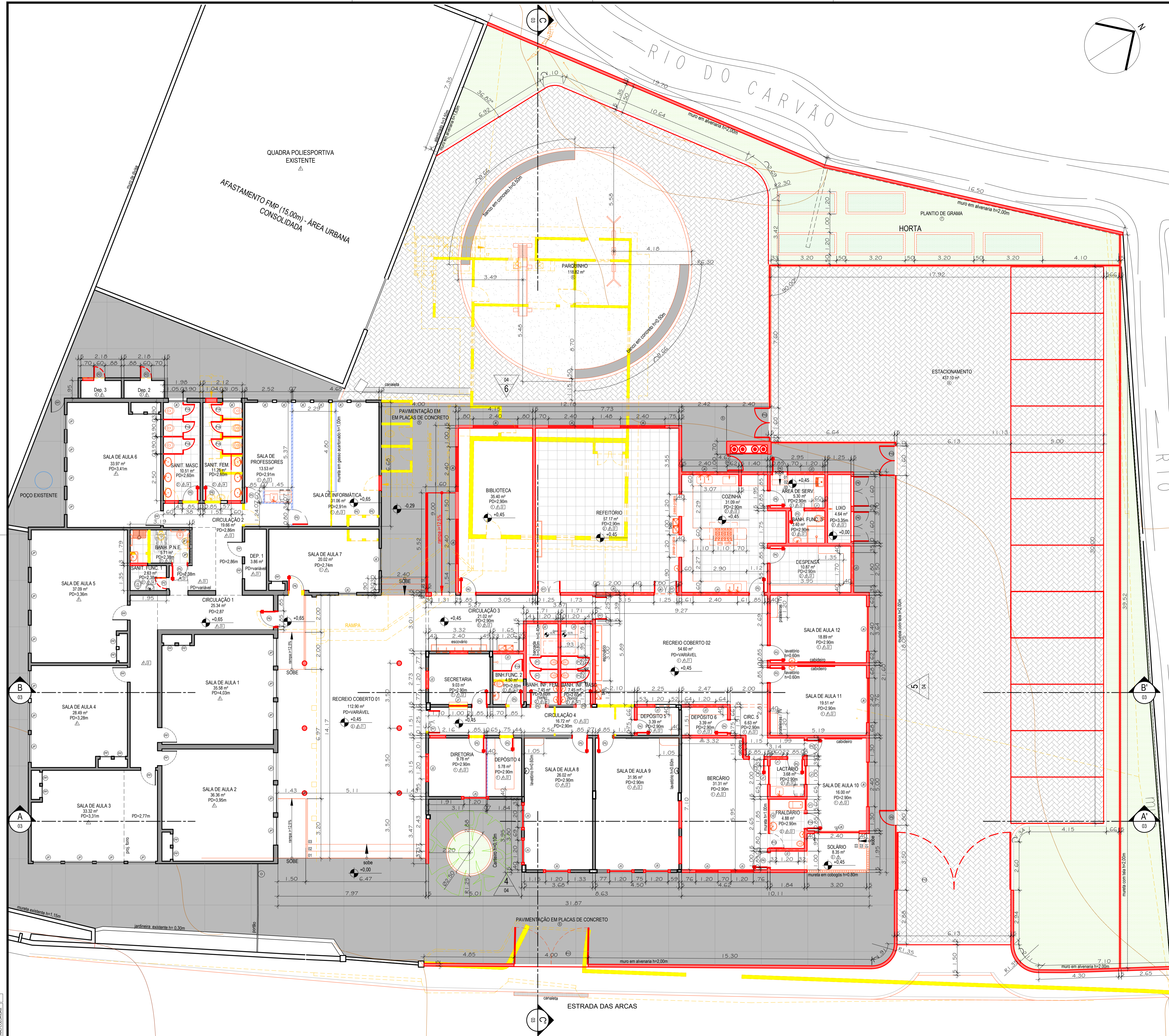
1 PLANTA BAIXA - DEMOLIR / CONSTRUIR ESCALA 1/100
