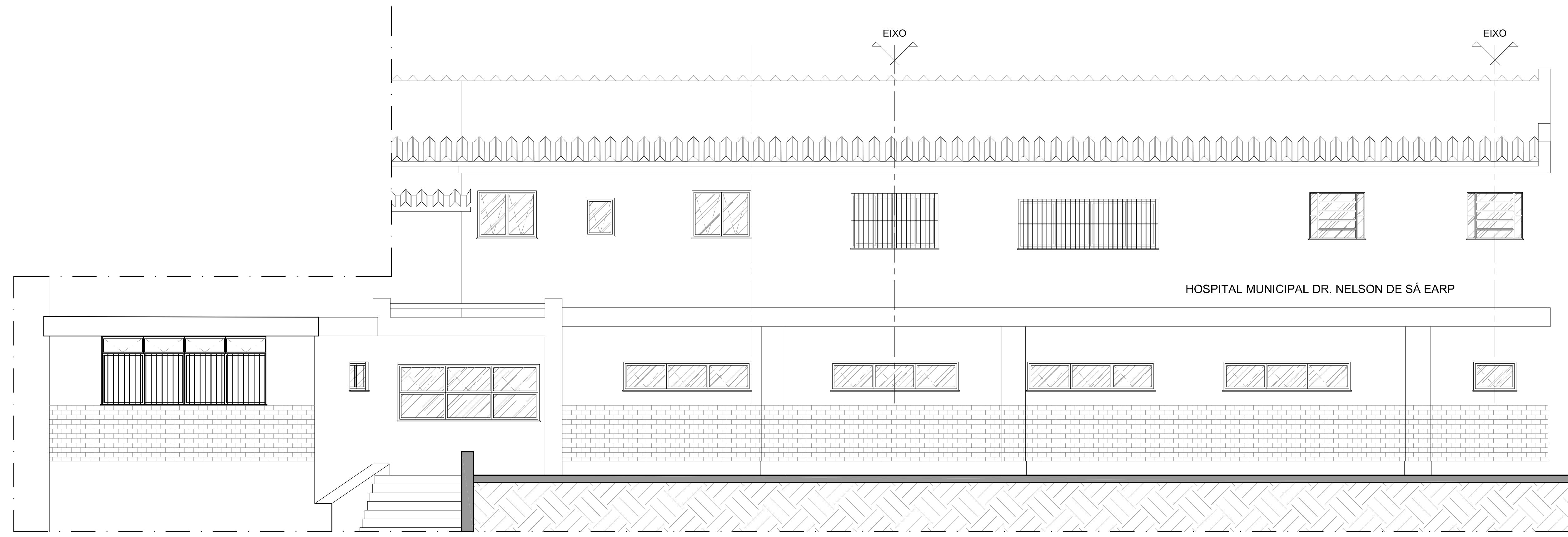
1 FACHADA PRINCIPAL esc.: 1/50
