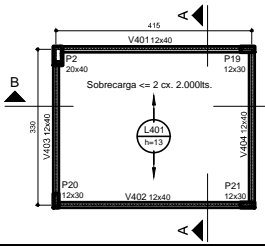
Forma do pavimento Piso Cx escala 1:50
