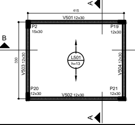
Forma do pavimento Teto Cx escala 1:50
