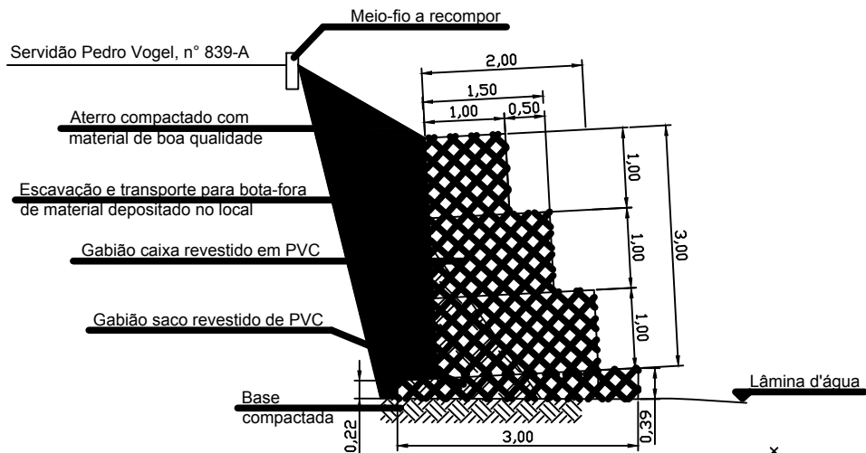
02 CORTE A-A' 1:75
