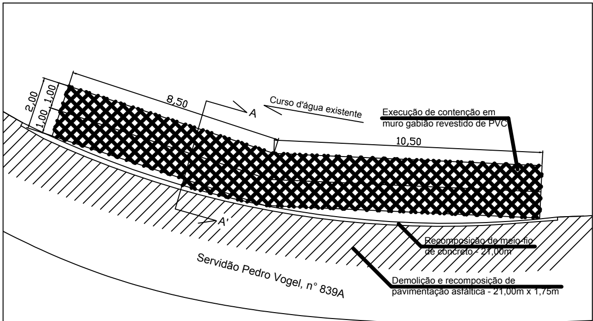
01 PLANTA BAIXA GERAL 1:125
