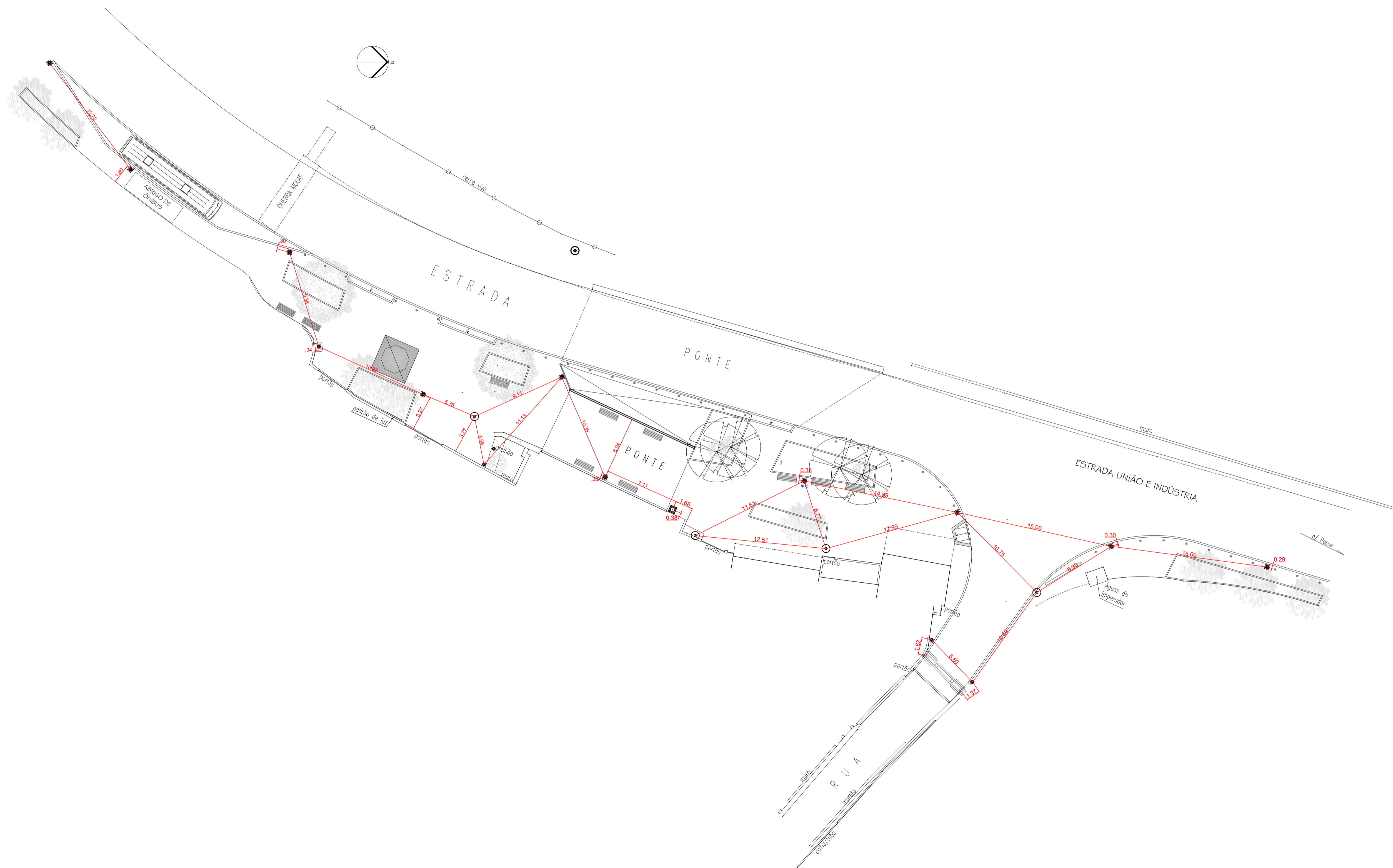
I PLANTA DE ILUMINAÇÃO PÚBLICA - LOCAÇÃO ESCALA 1/200 FASE II
