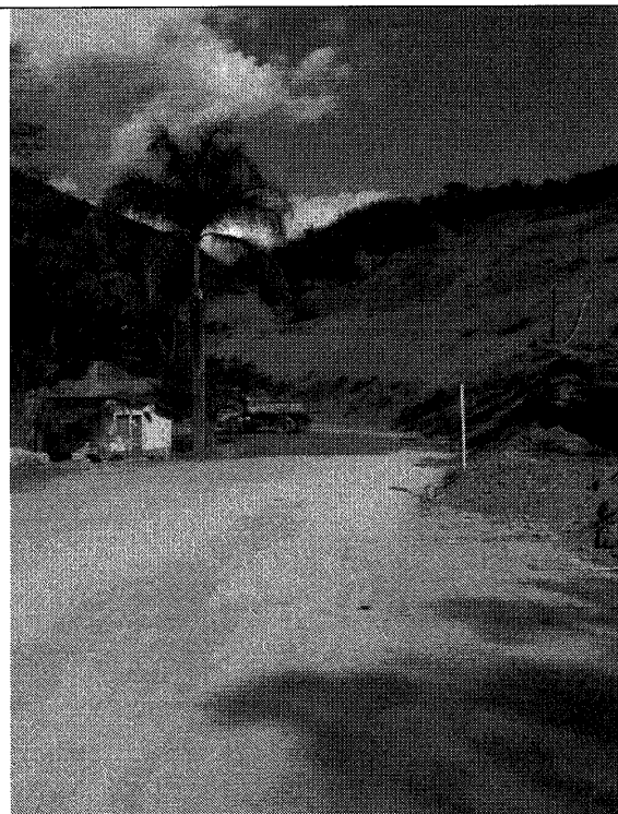
Área para a Implantação do Poço de Monitoramento PM2, Pé do Talude da Célula1
