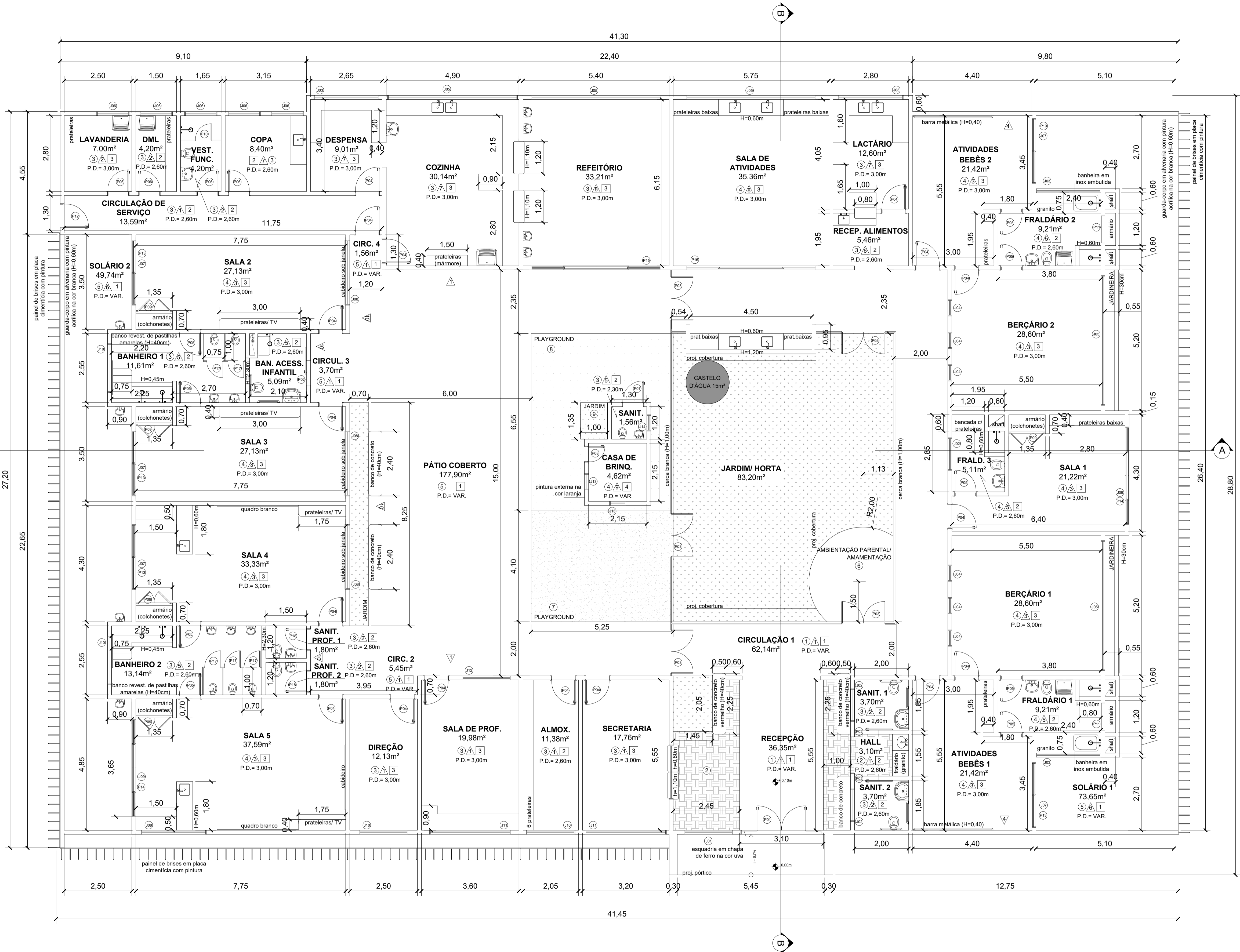
1 PLANTA BAIXA ESC.: 1/75
