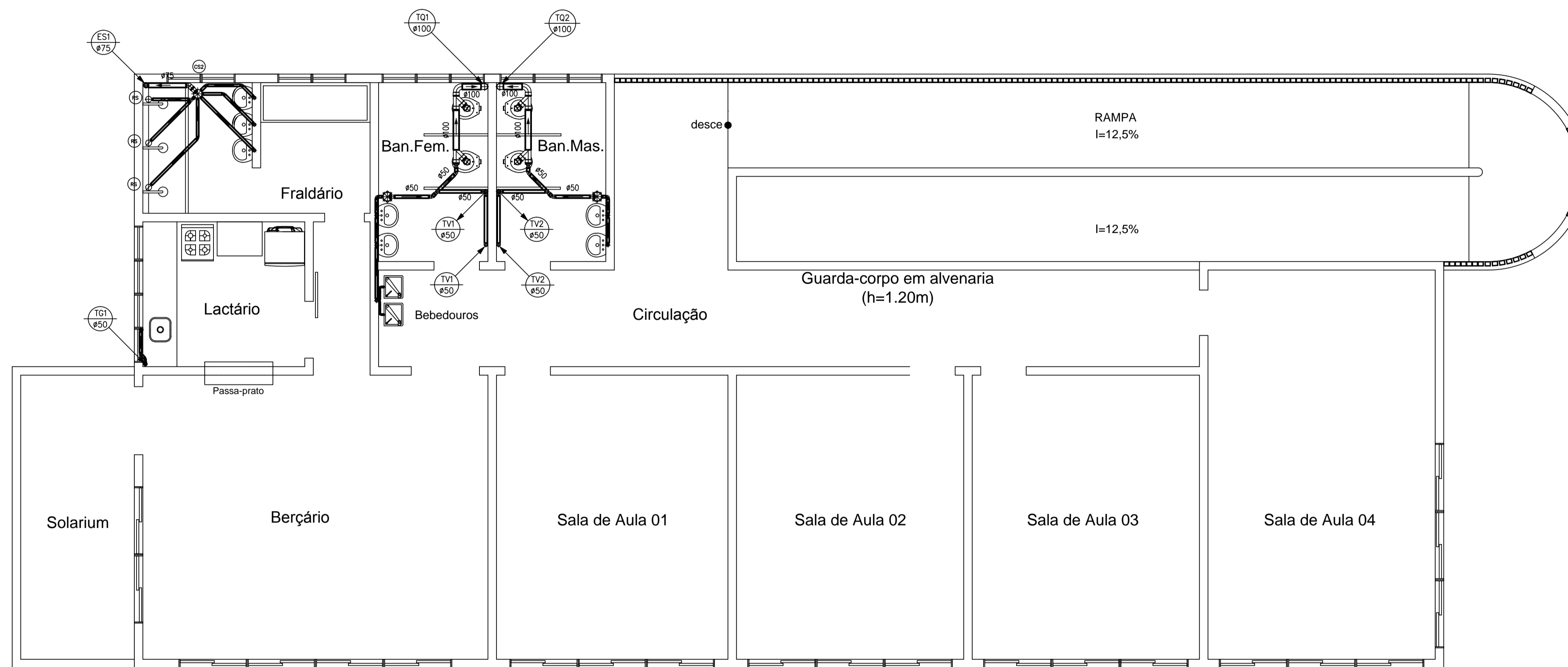
PLANTA BAIXA - SEGUNDO PAVIMENTO ESC. : 1/50
