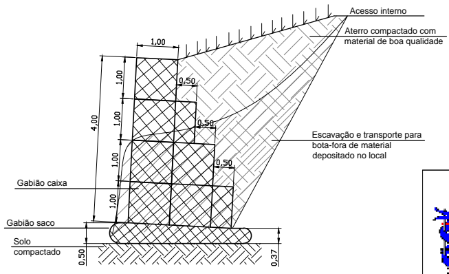
02 CORTE A-A' 1:125
