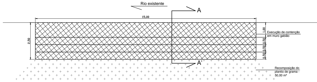
01 PLANTA BAIXA GERAL 1:125
