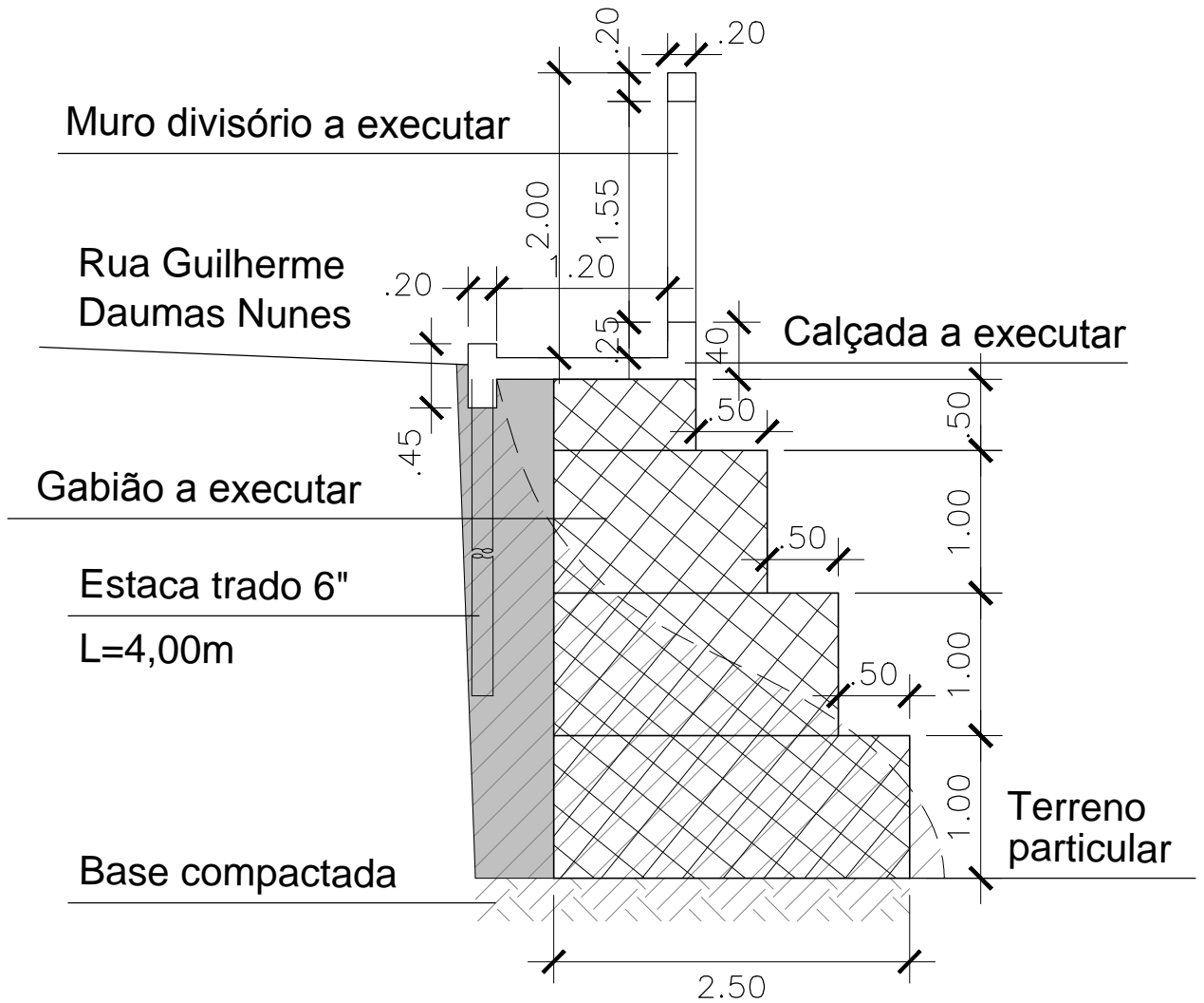
PERFIL A-A' 1:50
