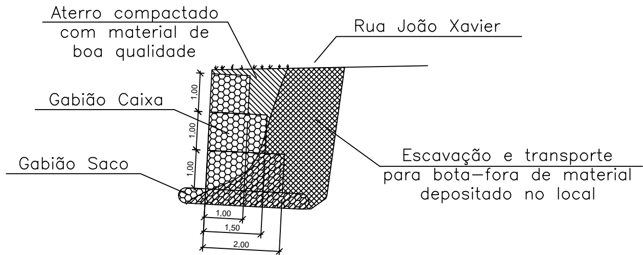
B CORTE A-A' Escala 1:100
