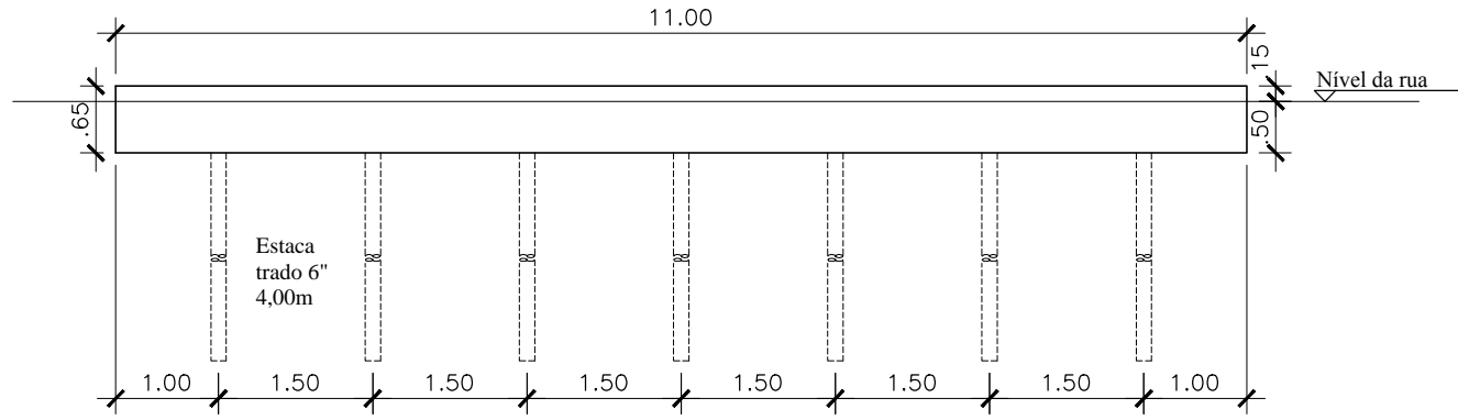
O1 DETALHE MEIO-FIO ESTAQUEADO 1:75
