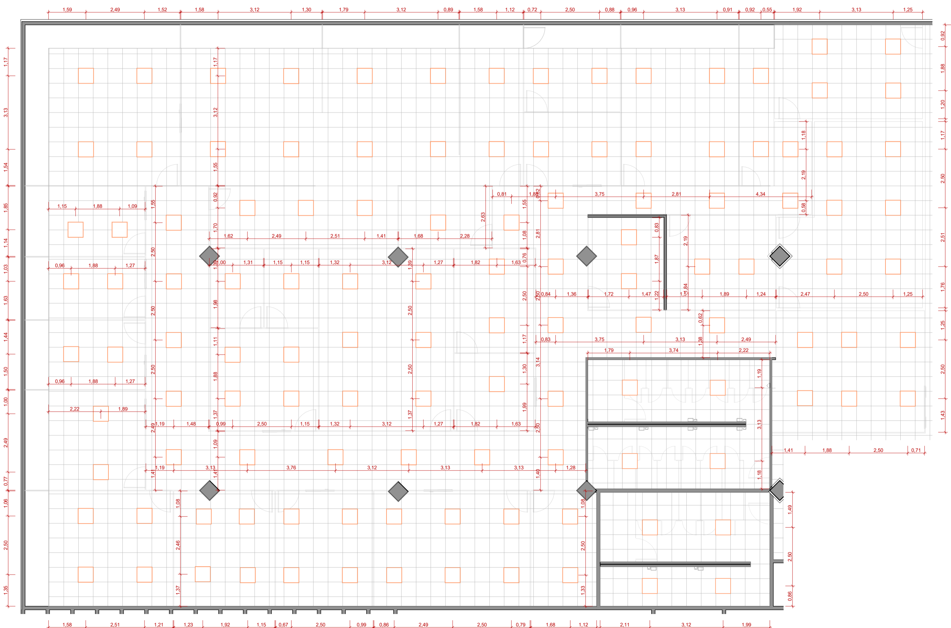
2 ILUMINAÇÃO ESC. 1 : 100
