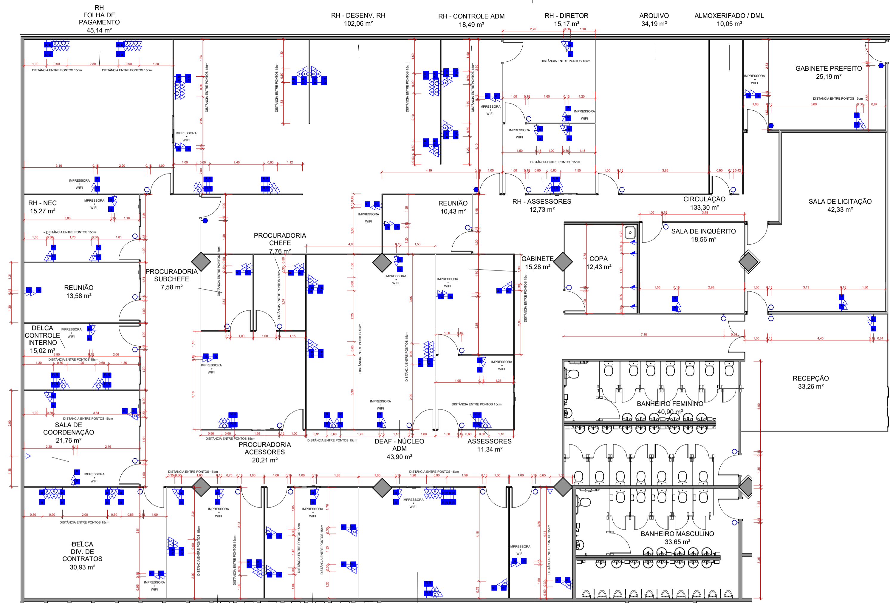
1 PONTOS ELÉTRICOS ESC. 1 : 100
