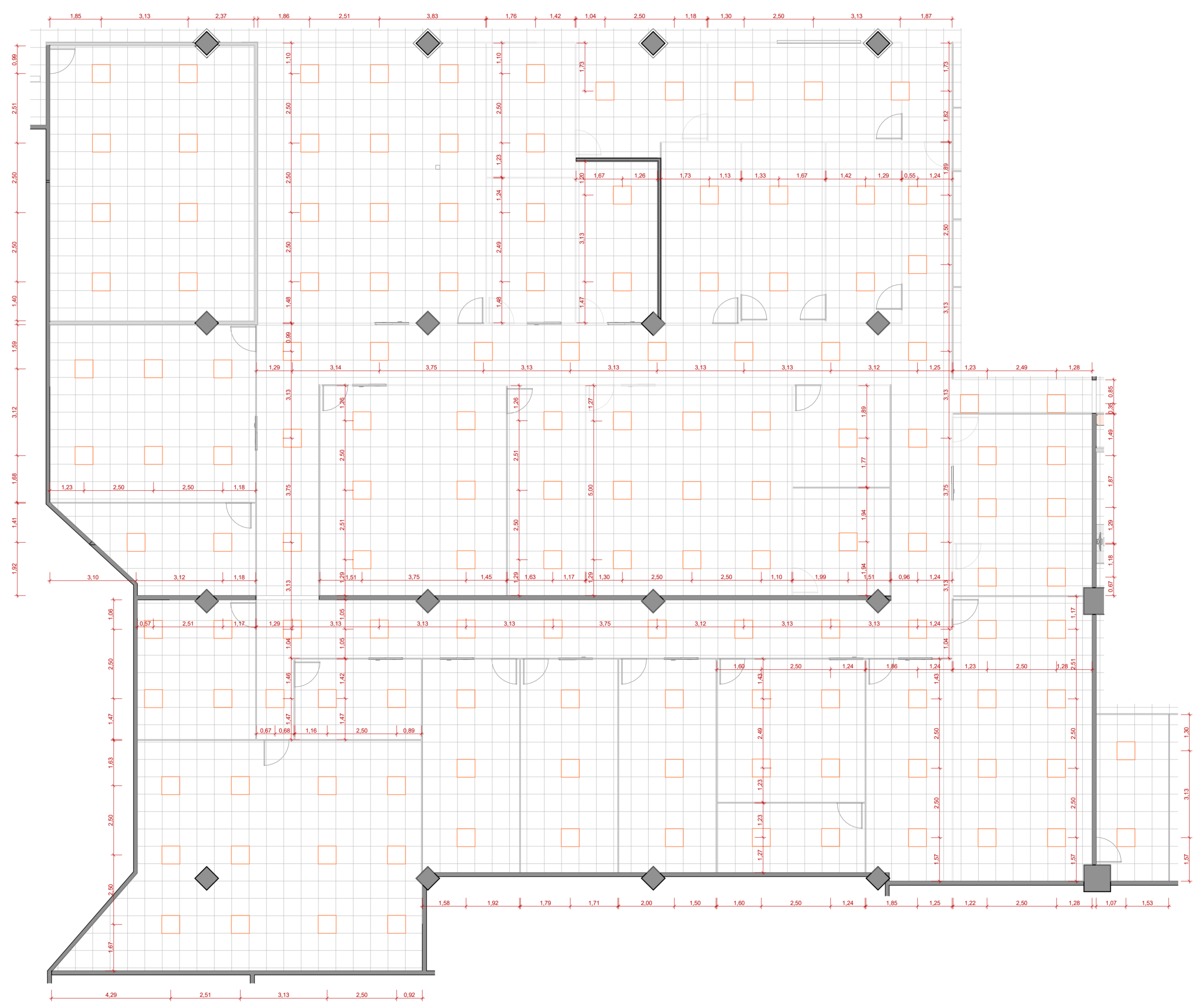
2 ILUMINAÇÃO ESC. 1 : 100
