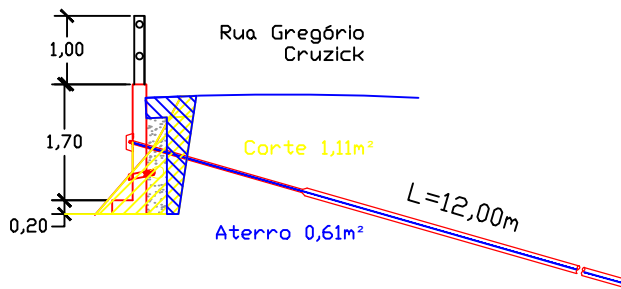
SEÇÃO C-C
