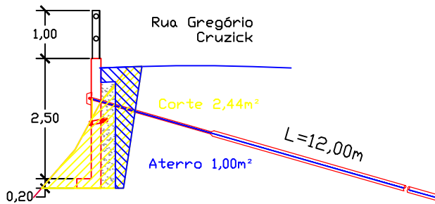
SEÇÃO B-B
