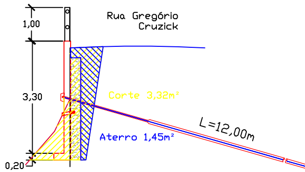
SEÇÃO A-A
