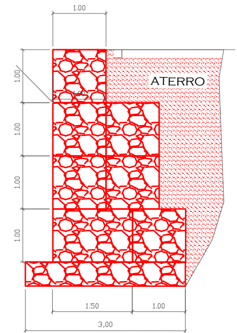
03 DETALHE 01 1:50
