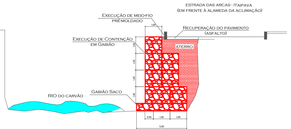
02 CORTE TRANSVERSAL 1:100
