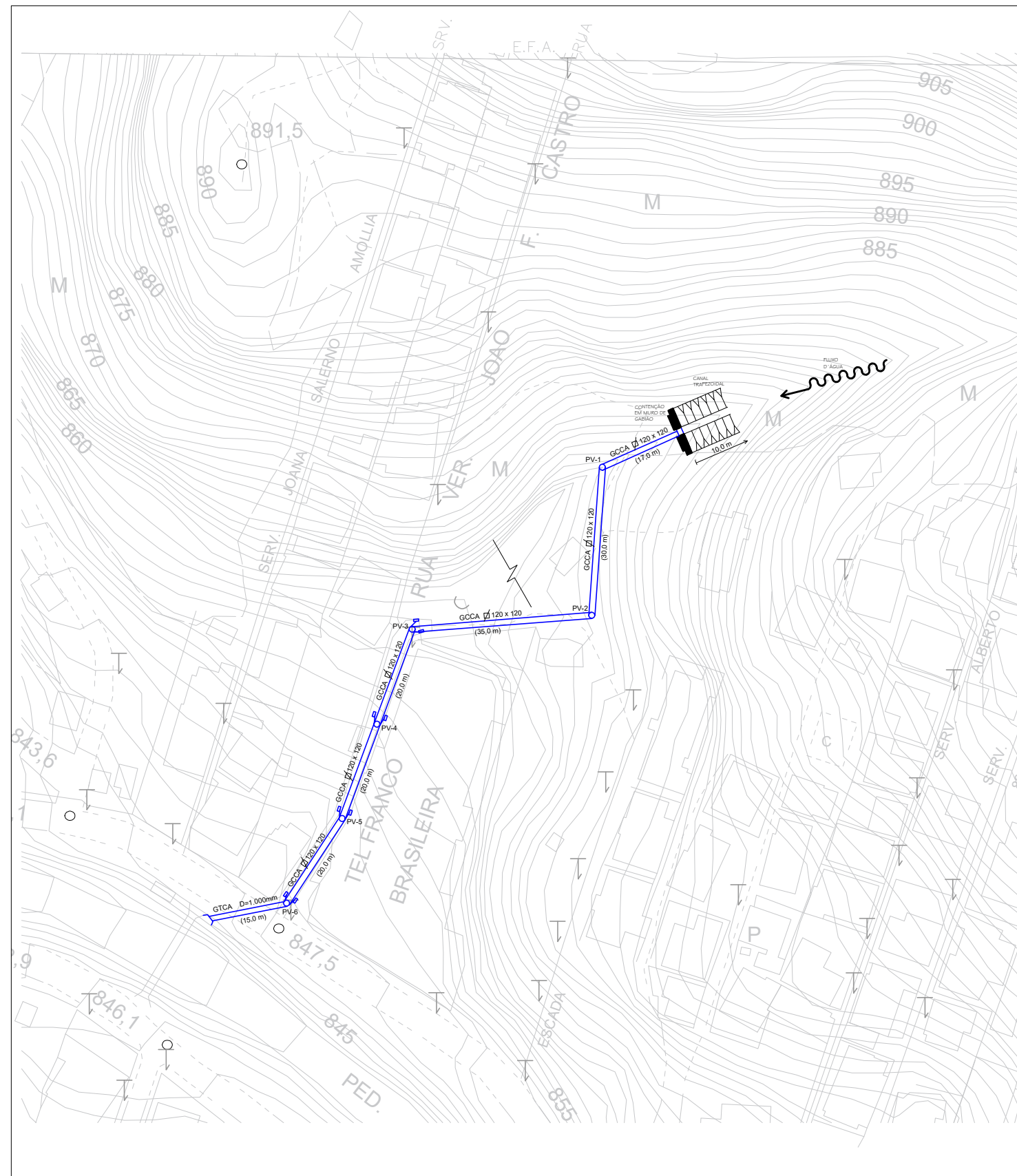
1 PLANTA DE IMPLANTAÇÃO ESCALA 1/500
