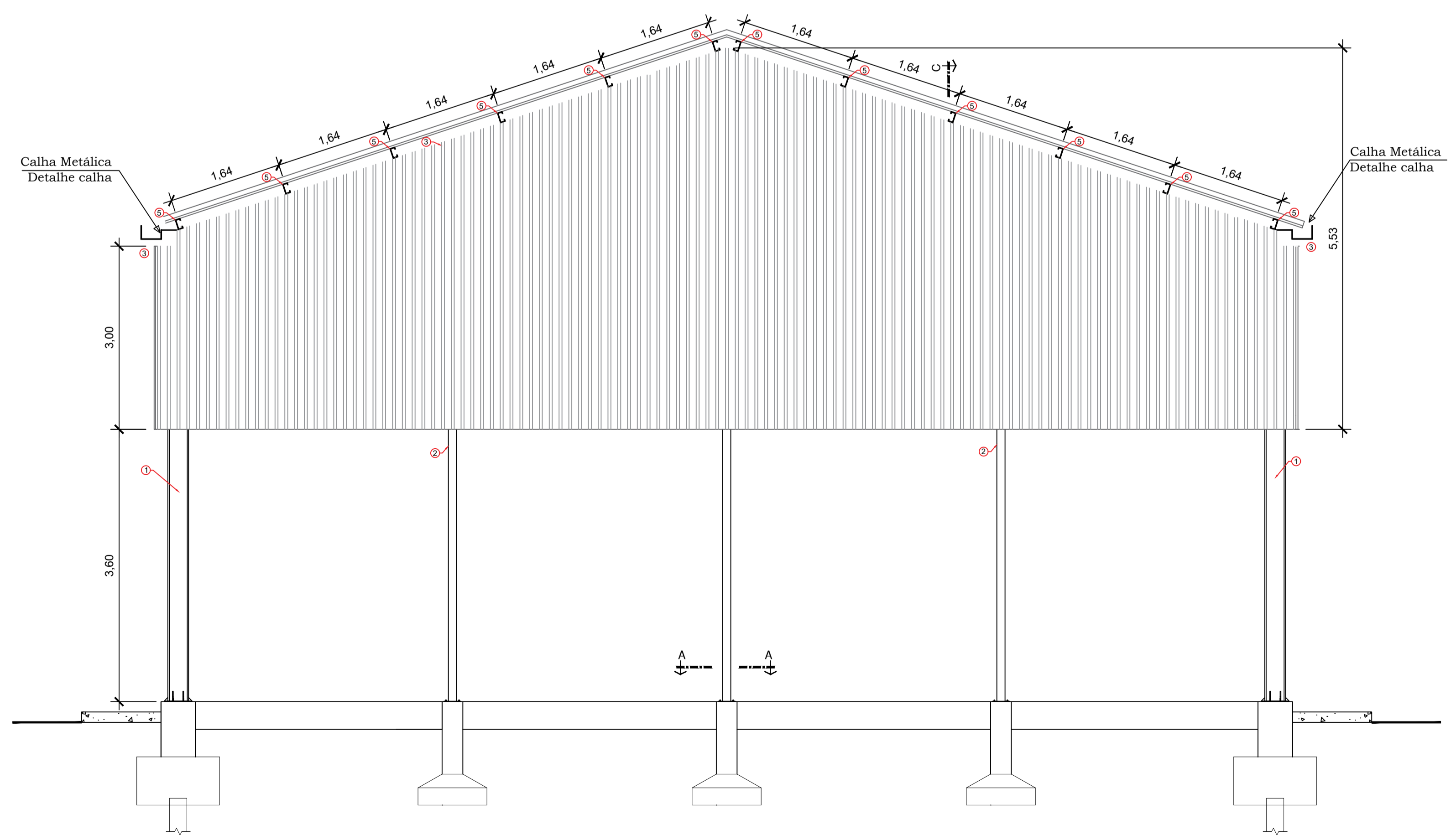
2 VISTA FRONTAL DA PLATIBANDA ESC: 1/50
