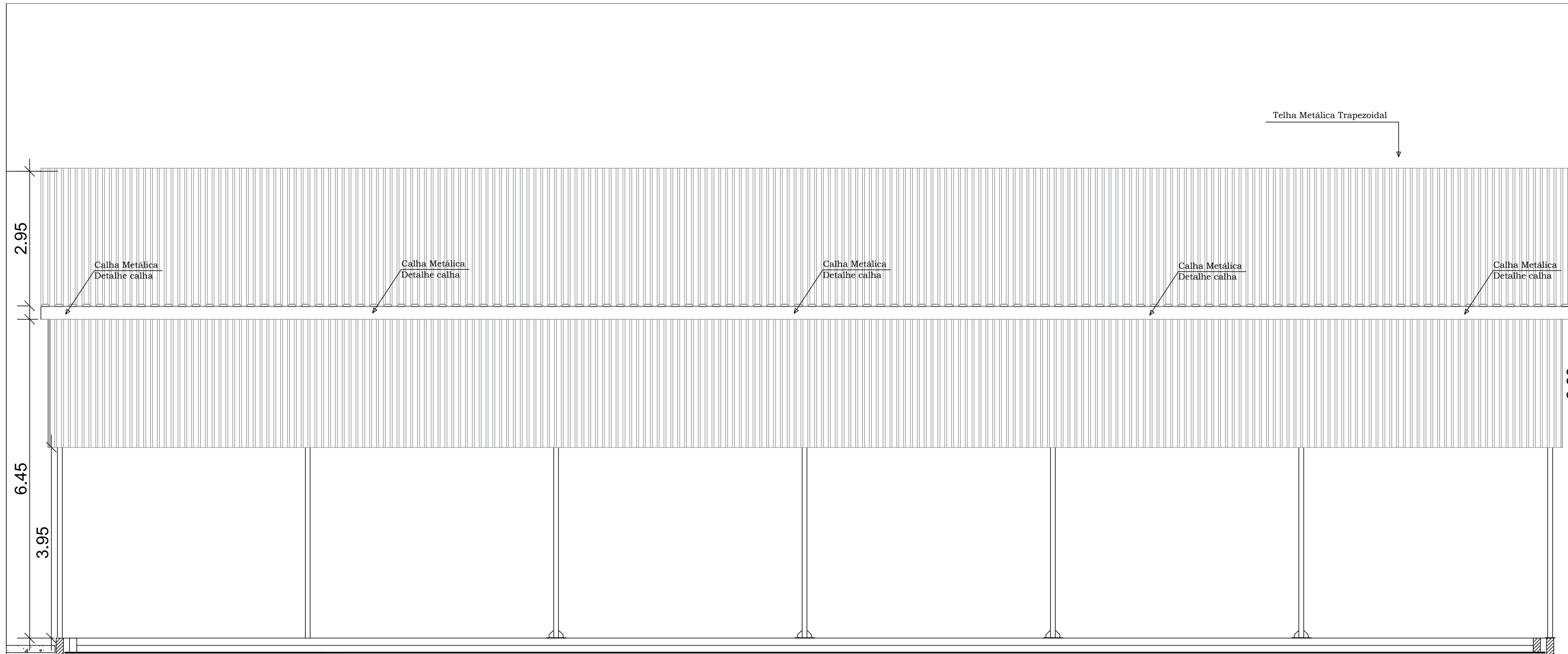
1 VISTA LATERAL DA PLATIBANDA ESC: 1/50
