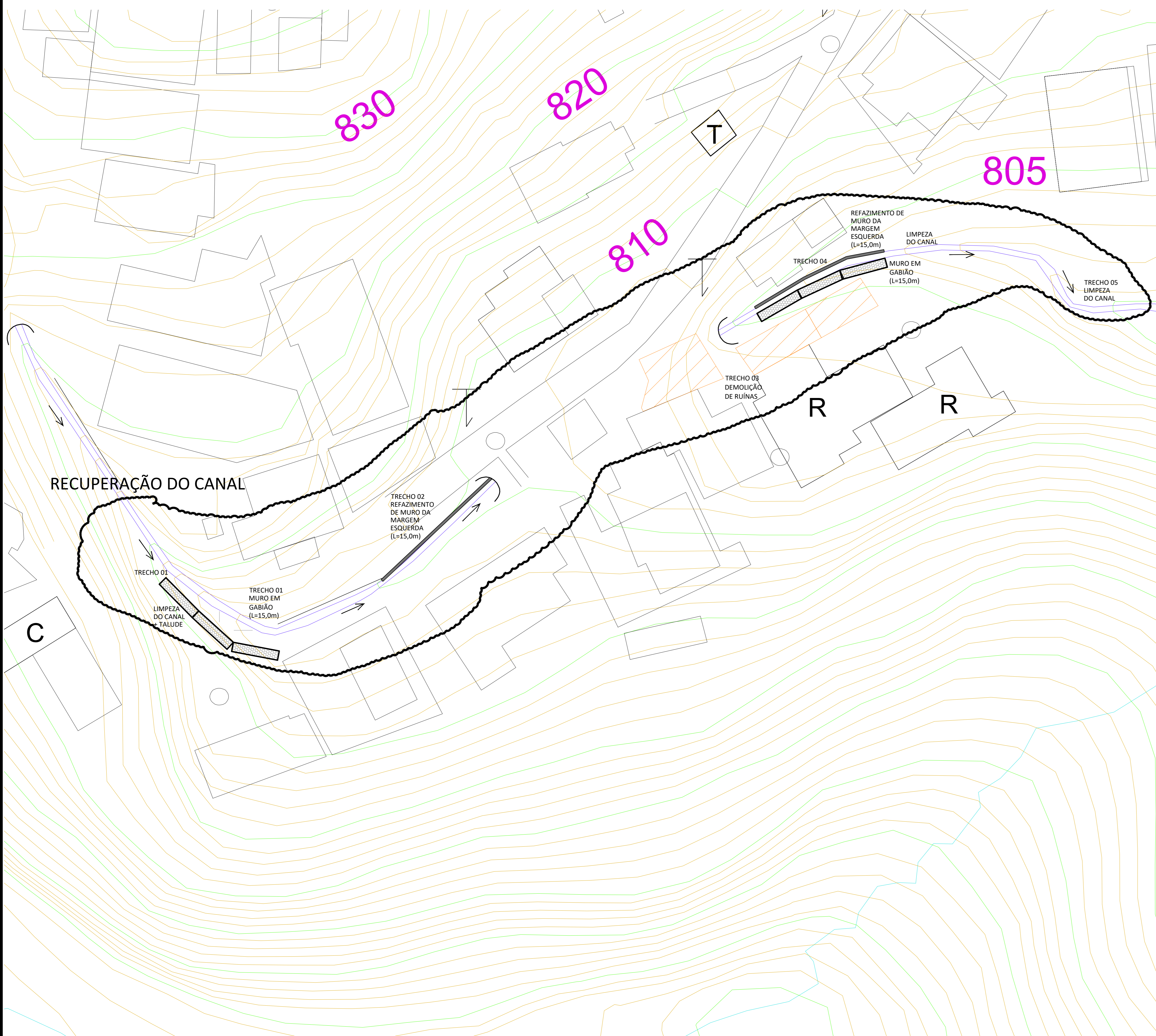
1 ARRANJO GERAL DE INTERVENÇÕES - TRAVESSA GOYTACAZES ESCALA 1/200
