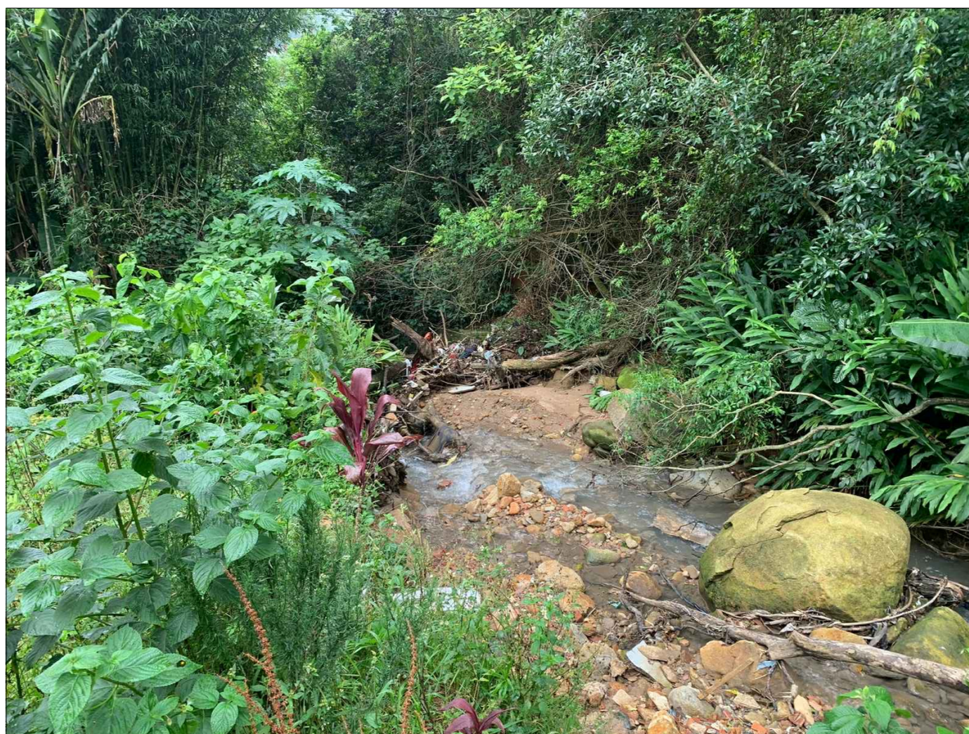
8 TRECHO 05 - LIMPEZA DO CANAL + REMOÇÃO DE BLOCOS DE ROCHA
