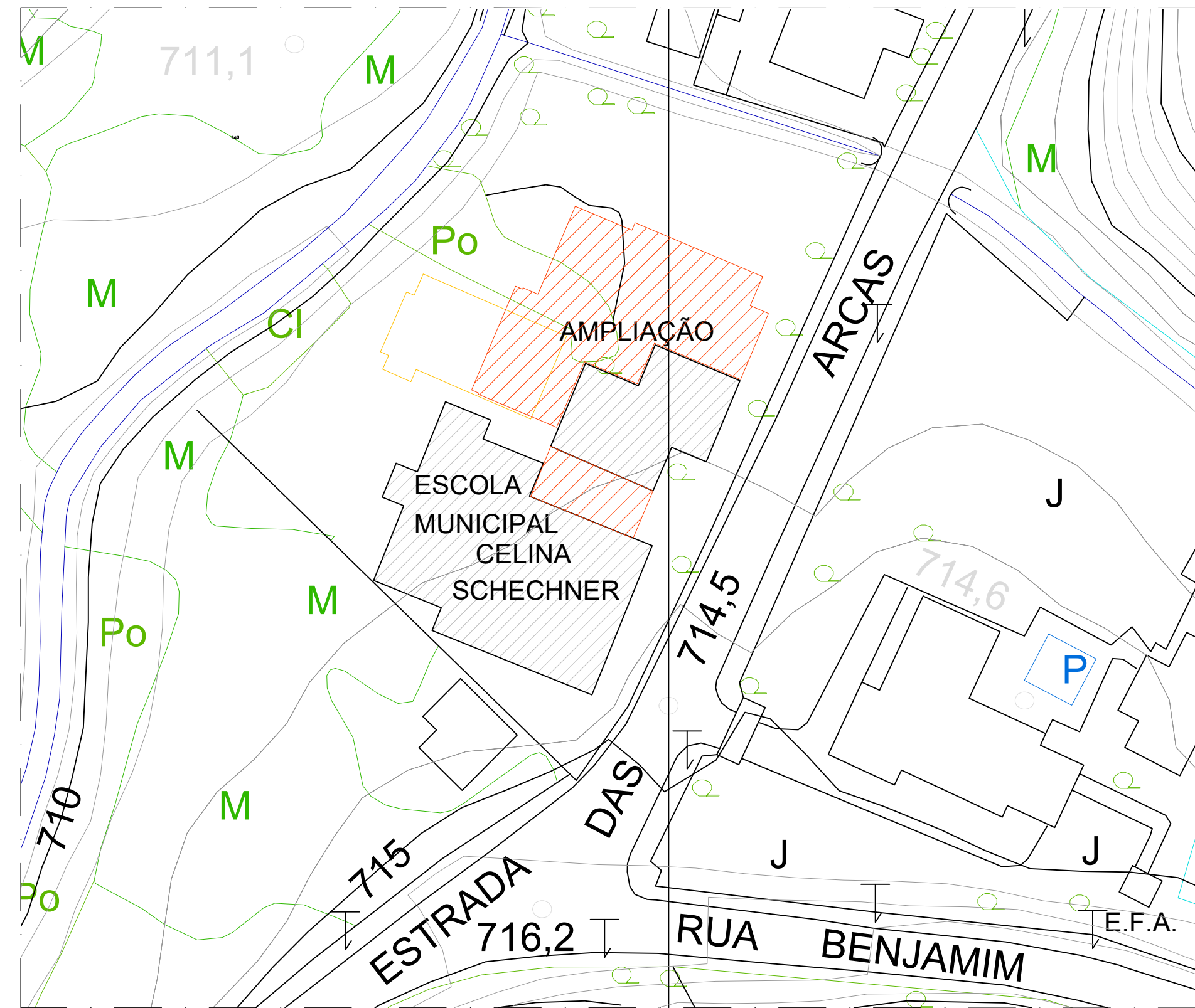
1 PLANTA DE SITUAÇÃO ESCALA 1/500
