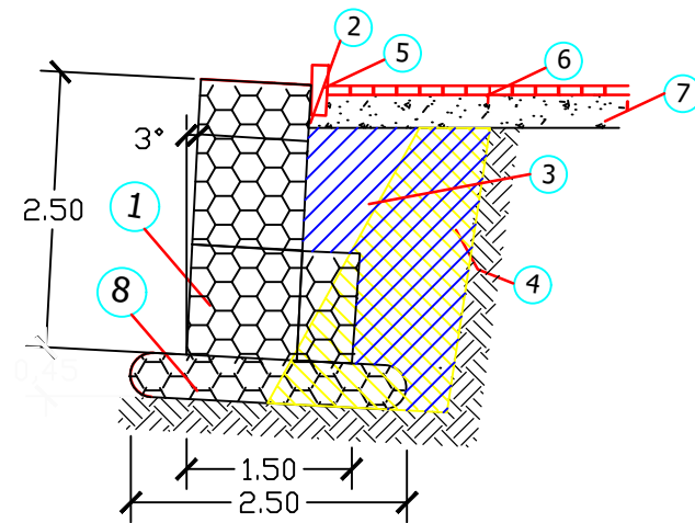
SEÇÃO TRANSVERSAL
