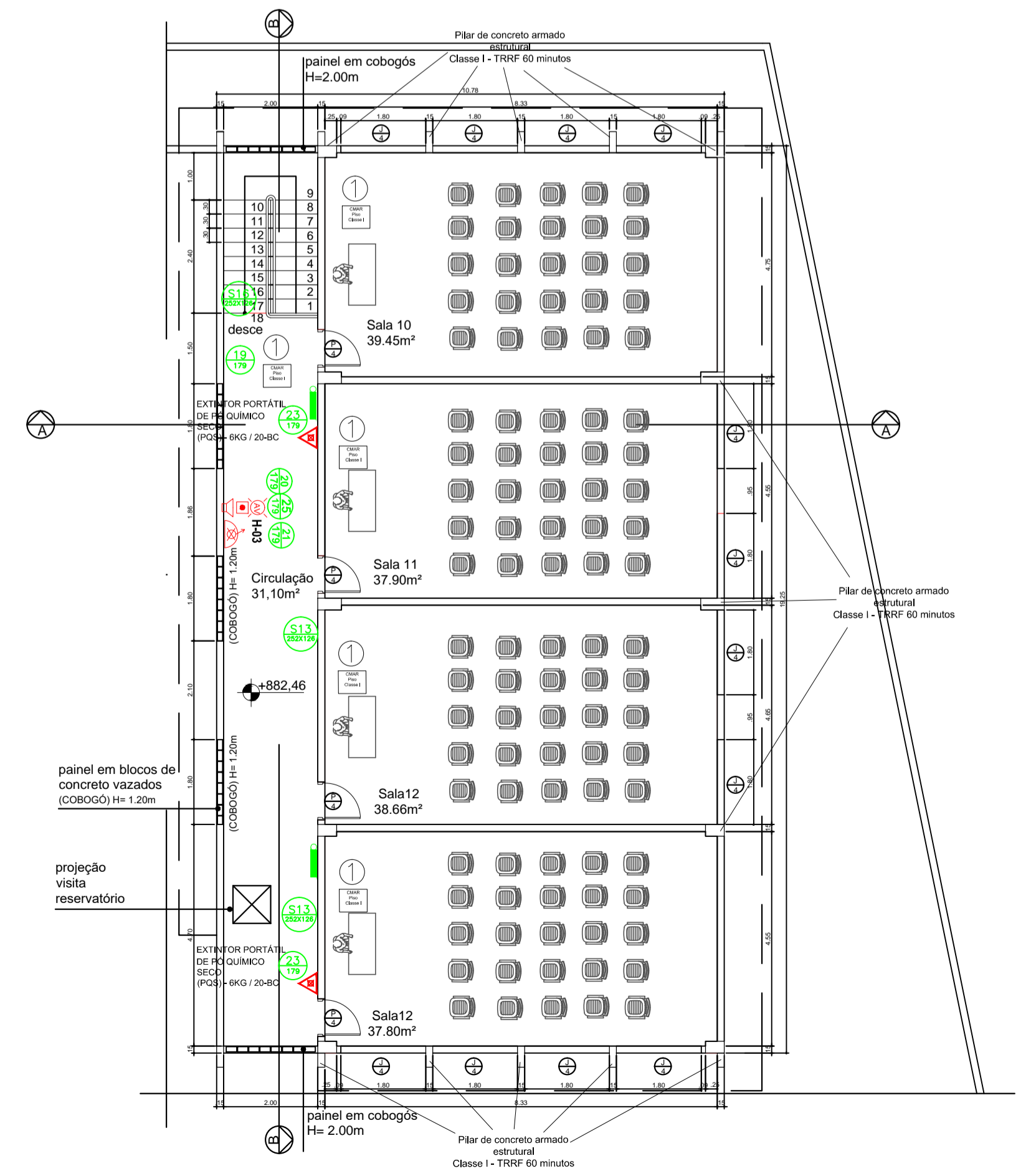
4 PLANTA BAIXA 2º PAVTO ESCALA: 1/100
