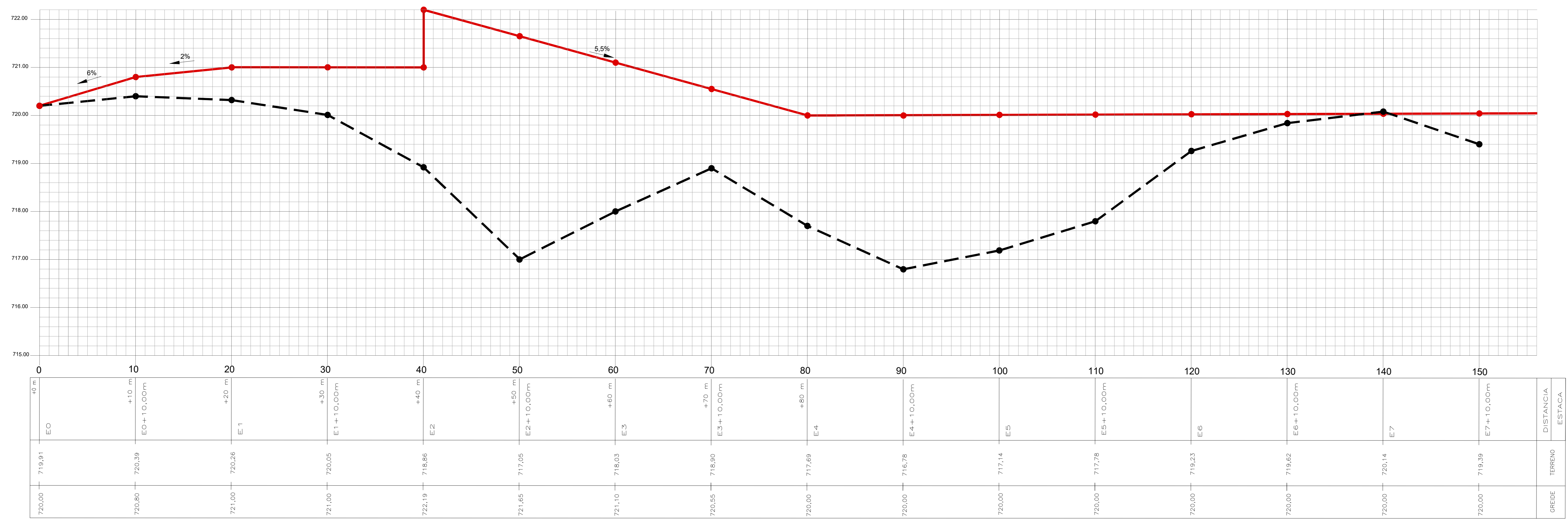
2 PERFIL DE GREIDE ESTACAS E0 A E7+10,00m 1/200
