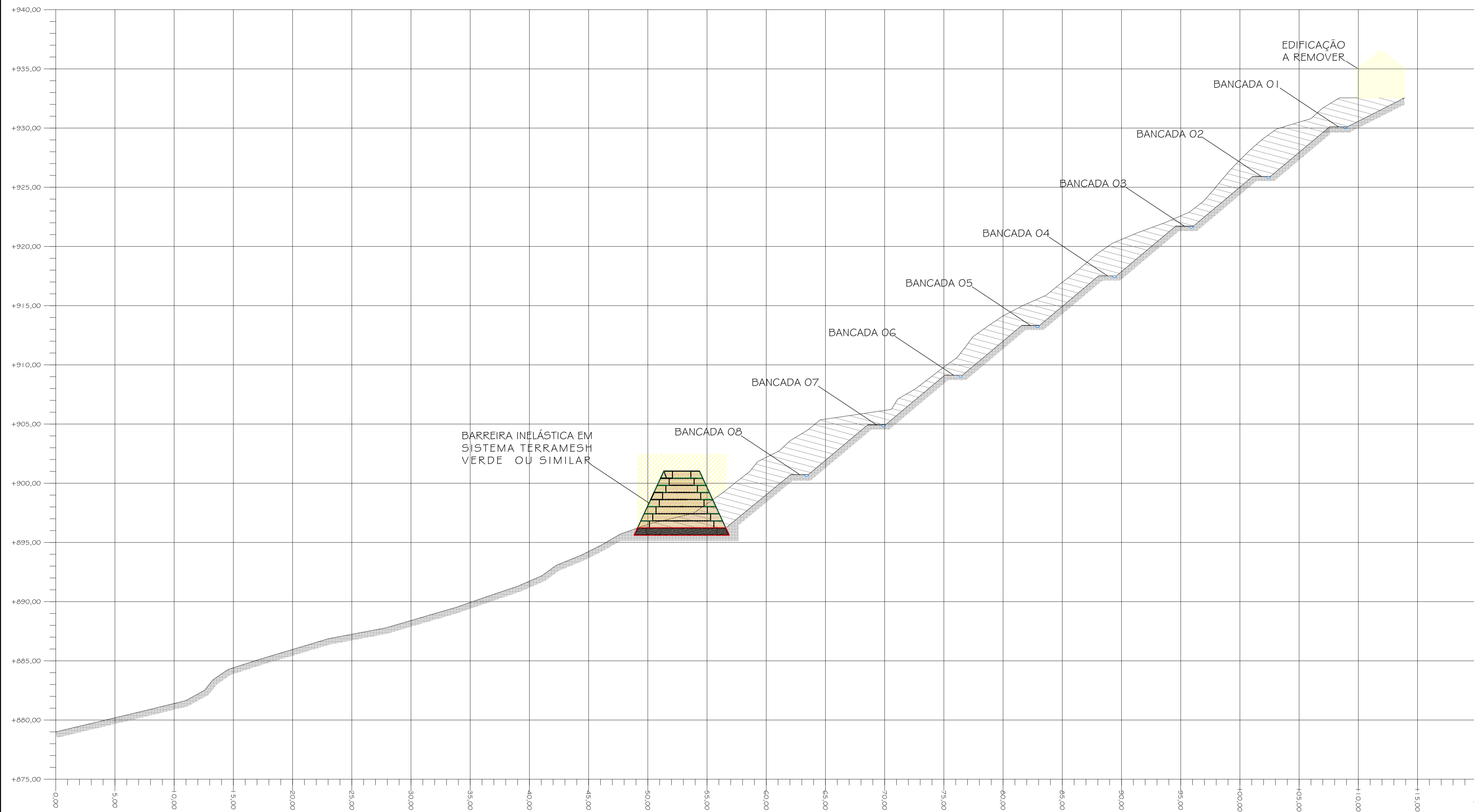
1 PERFIL LONGITUDINAL TALUDE 1/200
