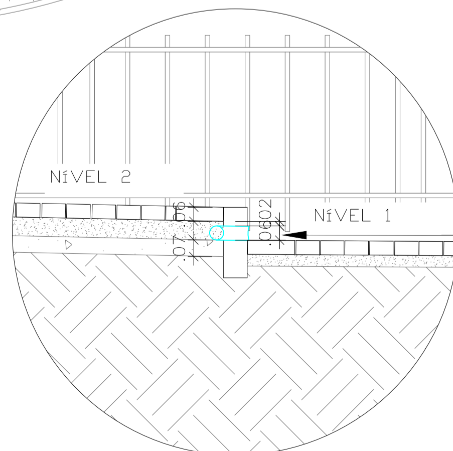
3 DETALHAM. DRENO CORTE S/ESC.
