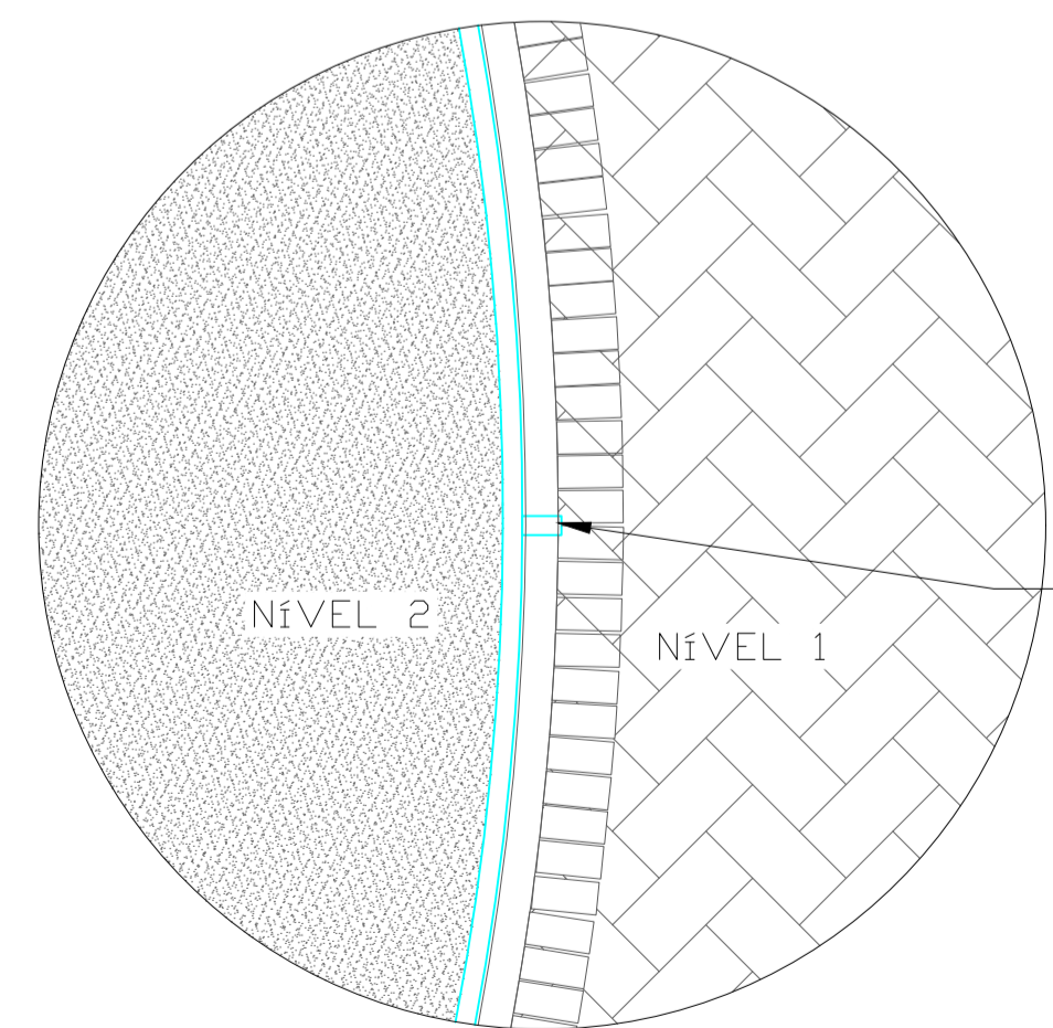
4 DETALHAM. DRENO NOS NÍVEIS S/ESC.
