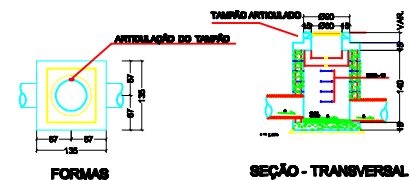
ESC. : 1/80 Cotas em centímetros
