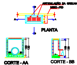
CORTE - AA ESC. : 1/80 Cotas em centímetros
