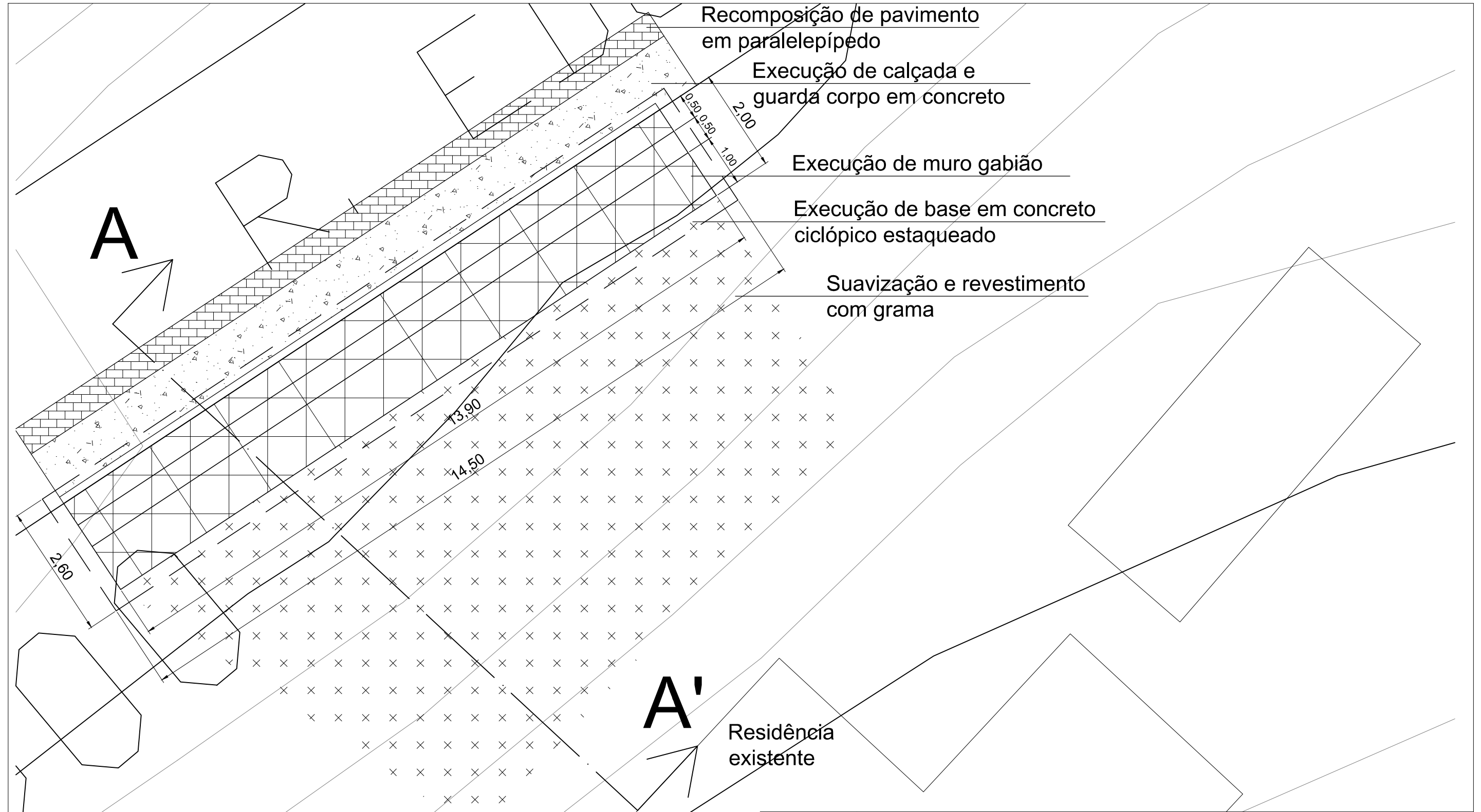
01 PLANTA BAIXA GERAL 1:75
