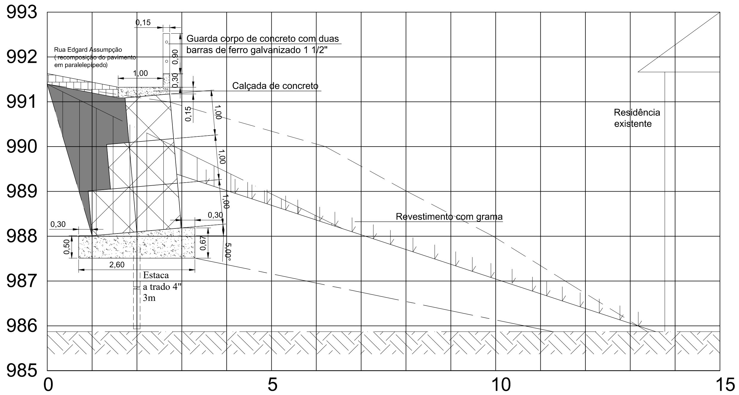
01 Corte A-A' 1:75
