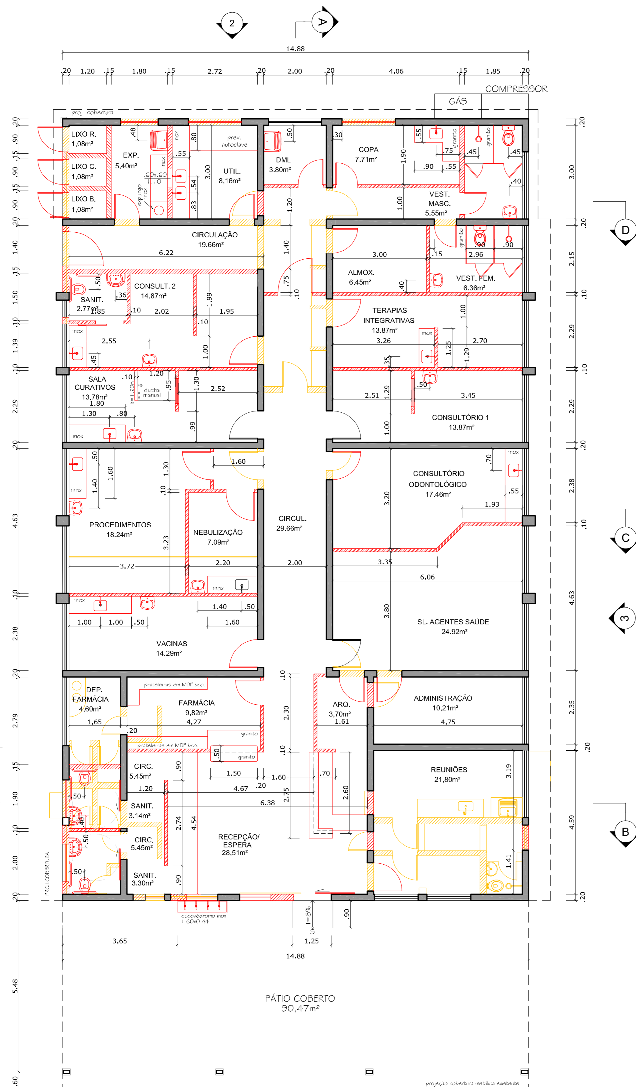
1 PLANTA DEMOLIR E CONSTRUIR esc: 1/75
