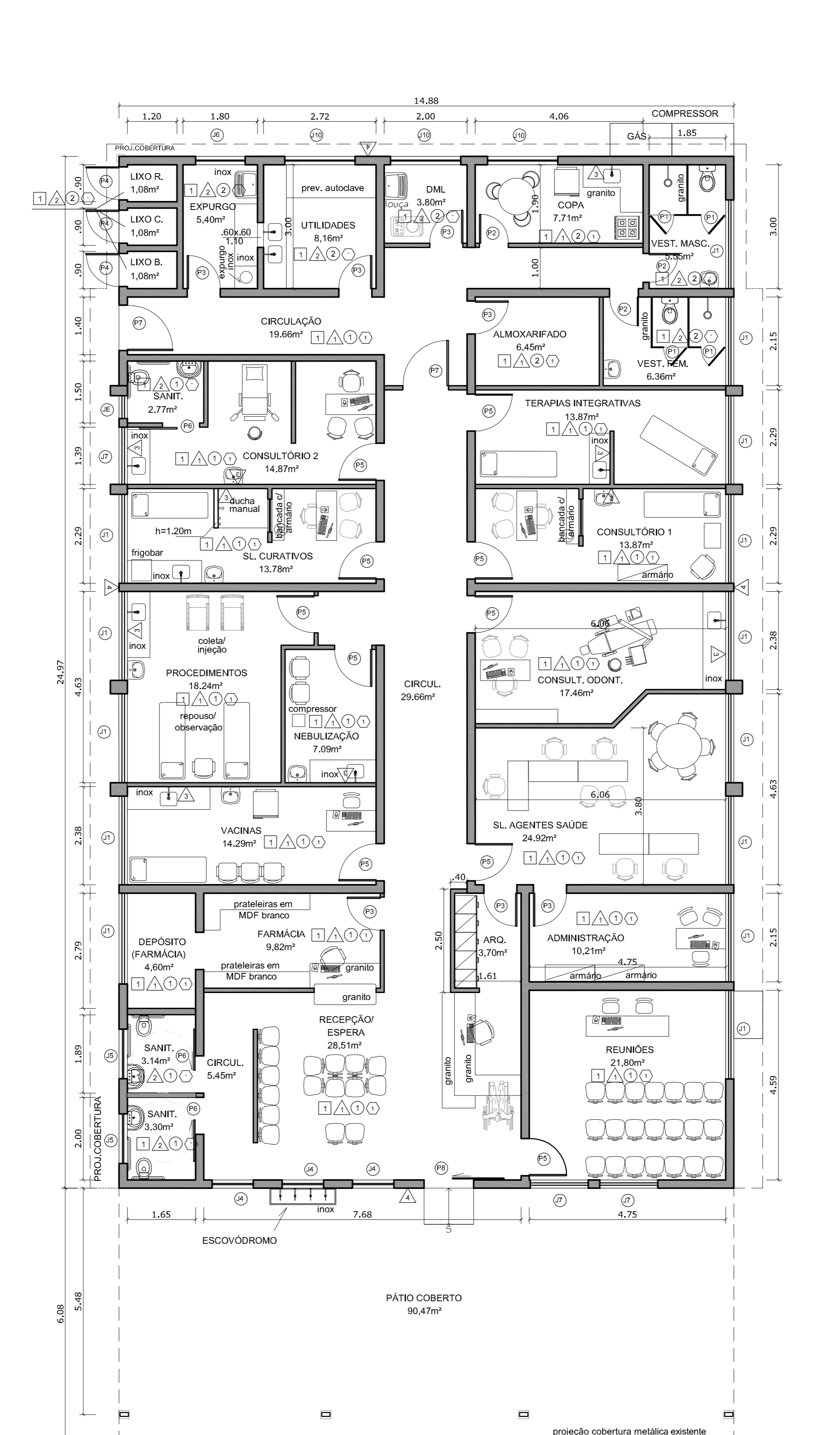
2 PLANTA DE ARQUITETURA esc: 1/75
