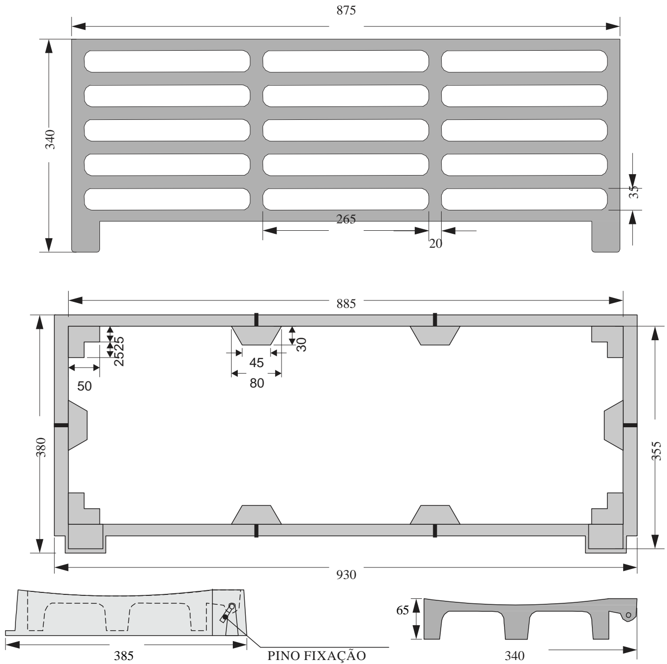
DETALHE SUPORTE
