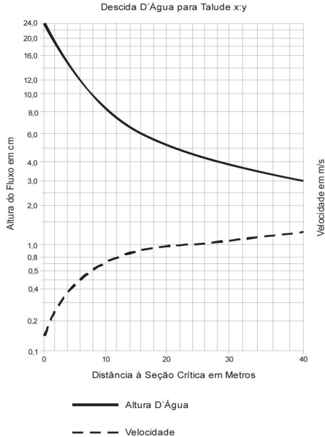
Figura - Curvas de profundidade e velocidade do líquido
