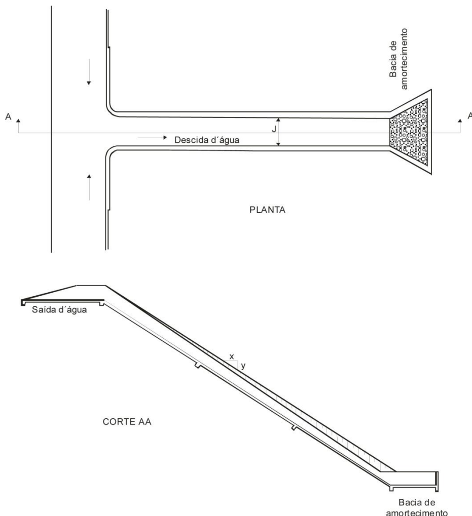
Figura – Descida d'água tipo rápido
