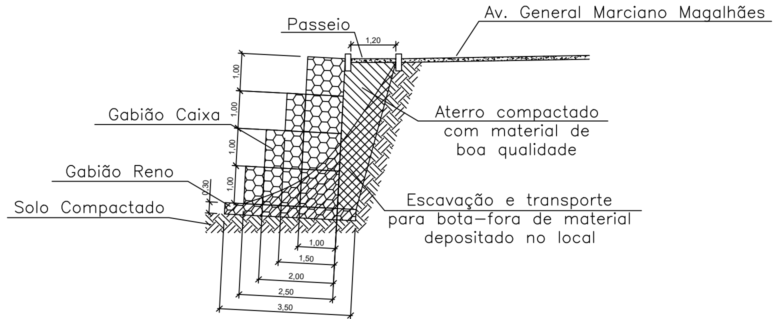
B CORTE A-A' Escala 1:100
