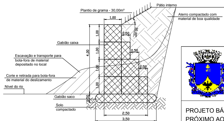
02 CORTE A-A' 1:125
