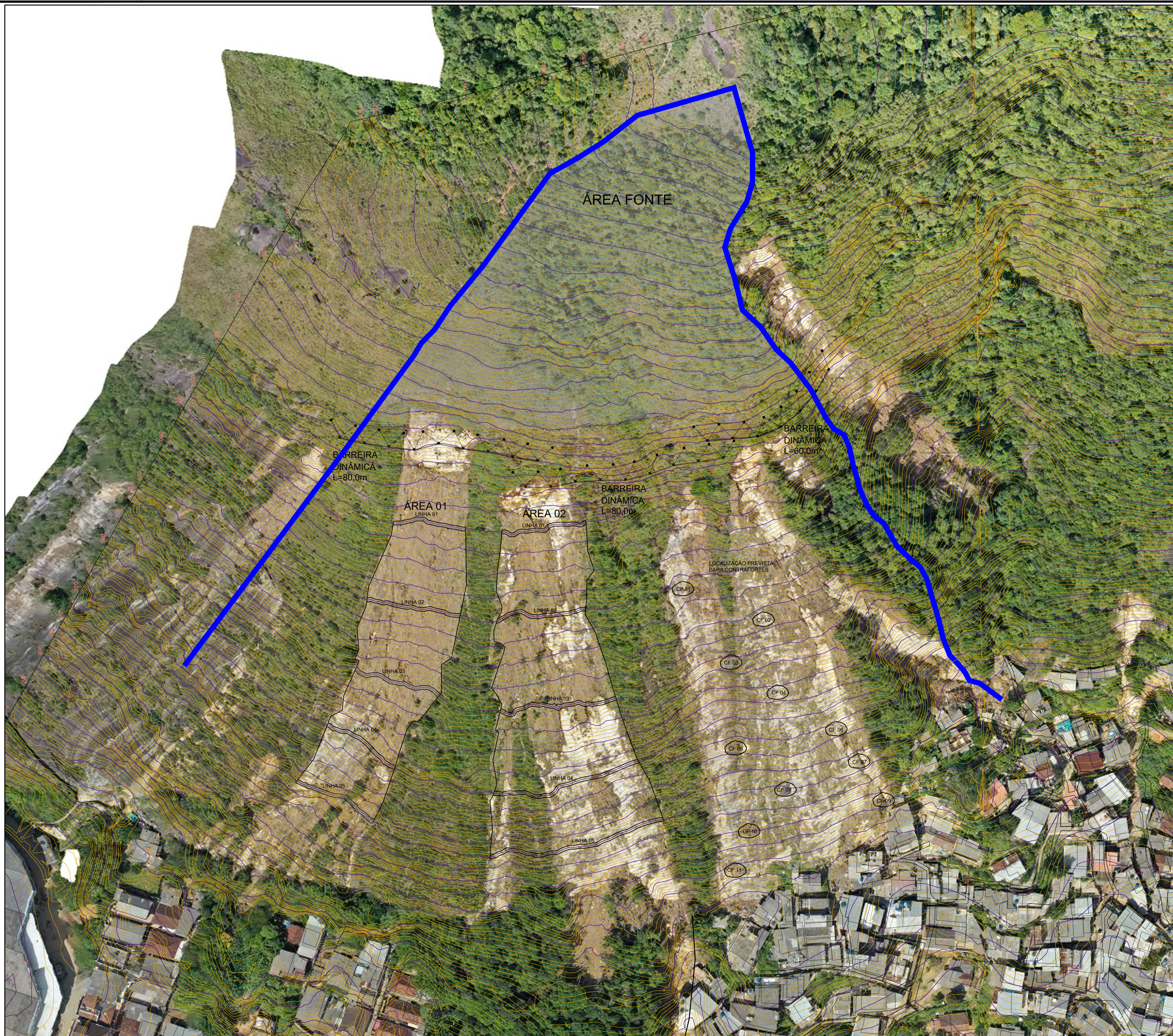
ARRANJO GERAL DE INTERVENÇÕES ESCALA 1/750
