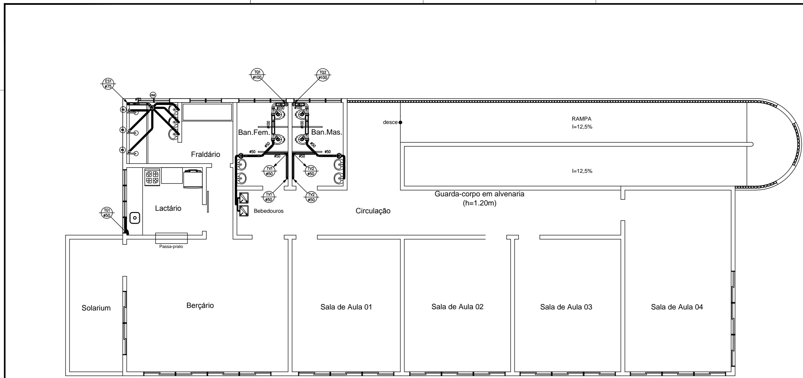
PLANTA BAIXA - SEGUNDO PAVIMENTO ESC. : 1/50
