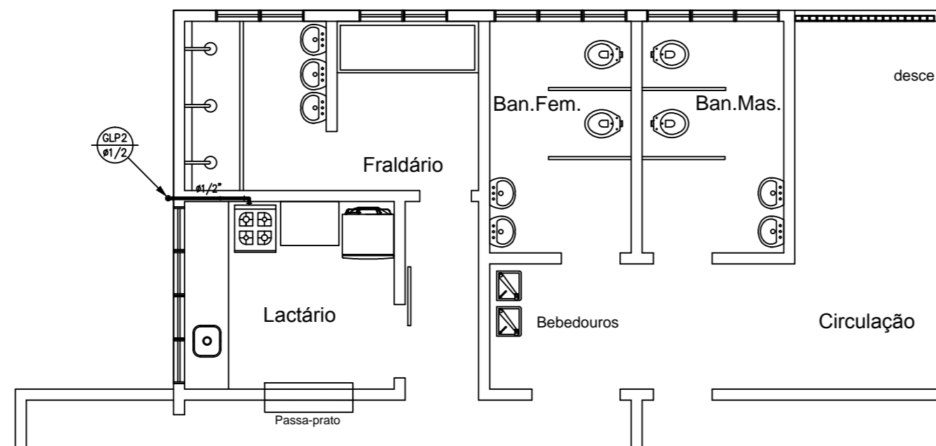
PLANTA BAIXA - SEGUNDO PAVIMENTO ESC.: 1/50
