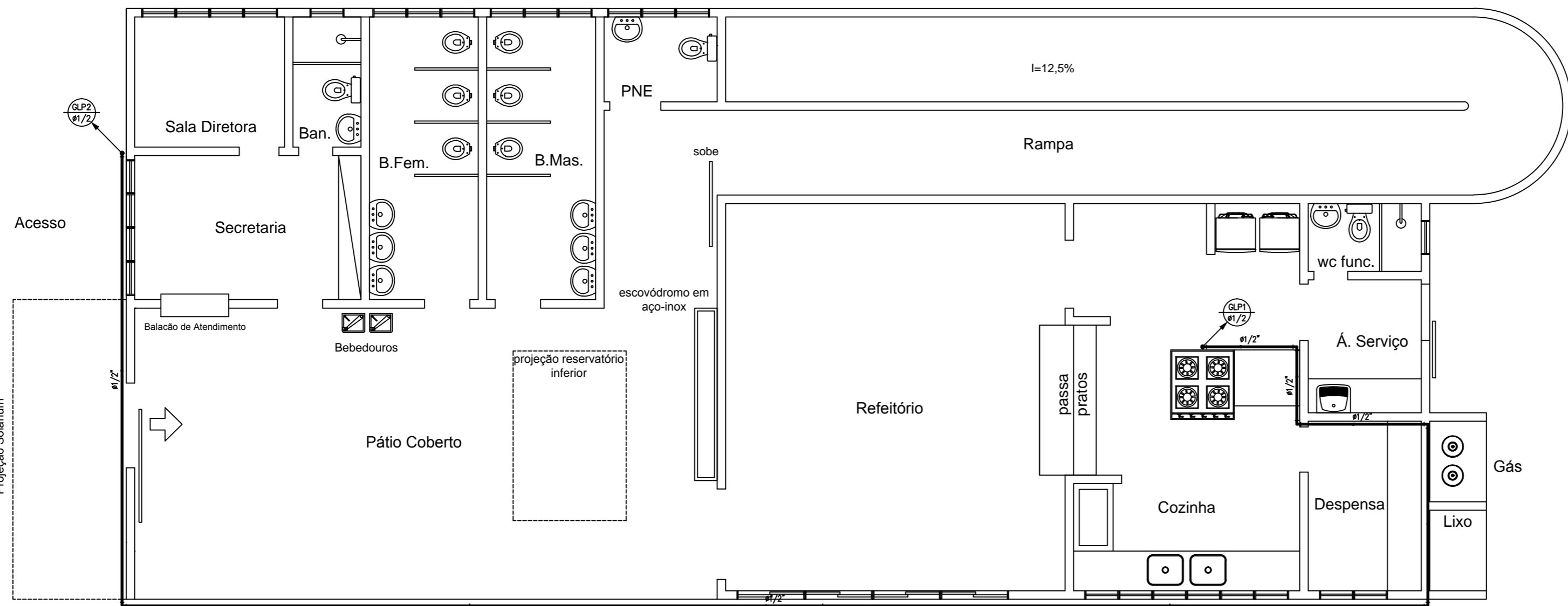
PLANTA BAIXA - PAVIMENTO TÉRREO ESC.: 1/50
