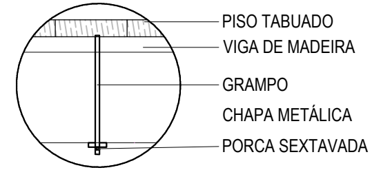
DETALHE 02 - GRAMPO E VIGA (ESC.: 1:20)
