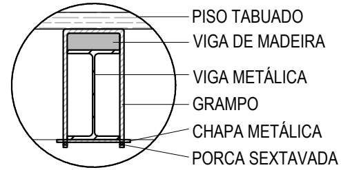
DETALHE 01 - GRAMPO E VIGA (ESC.: 1:20)
