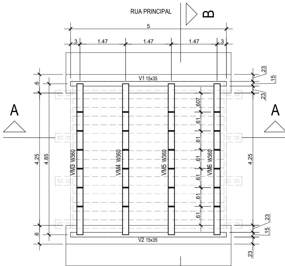
01 PL. BAIXA ESTRUTURA ESC.: 1/75
