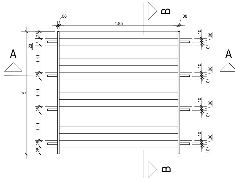
02 PL. BAIXA TABULEIRO ESC.: 1/75
