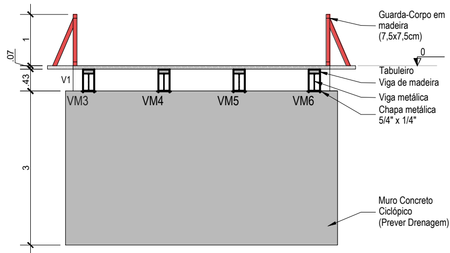
01 CORTE AA ESC.: 1/75
