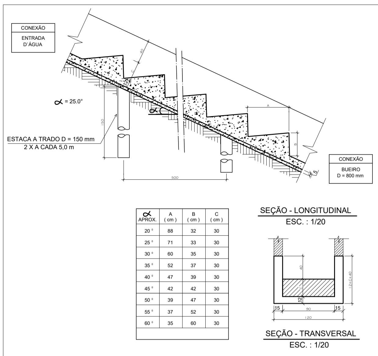
DAD 40x90 - SEÇÕES LONGITUDINAL E TRANSVERSAL SEM ESCALA
