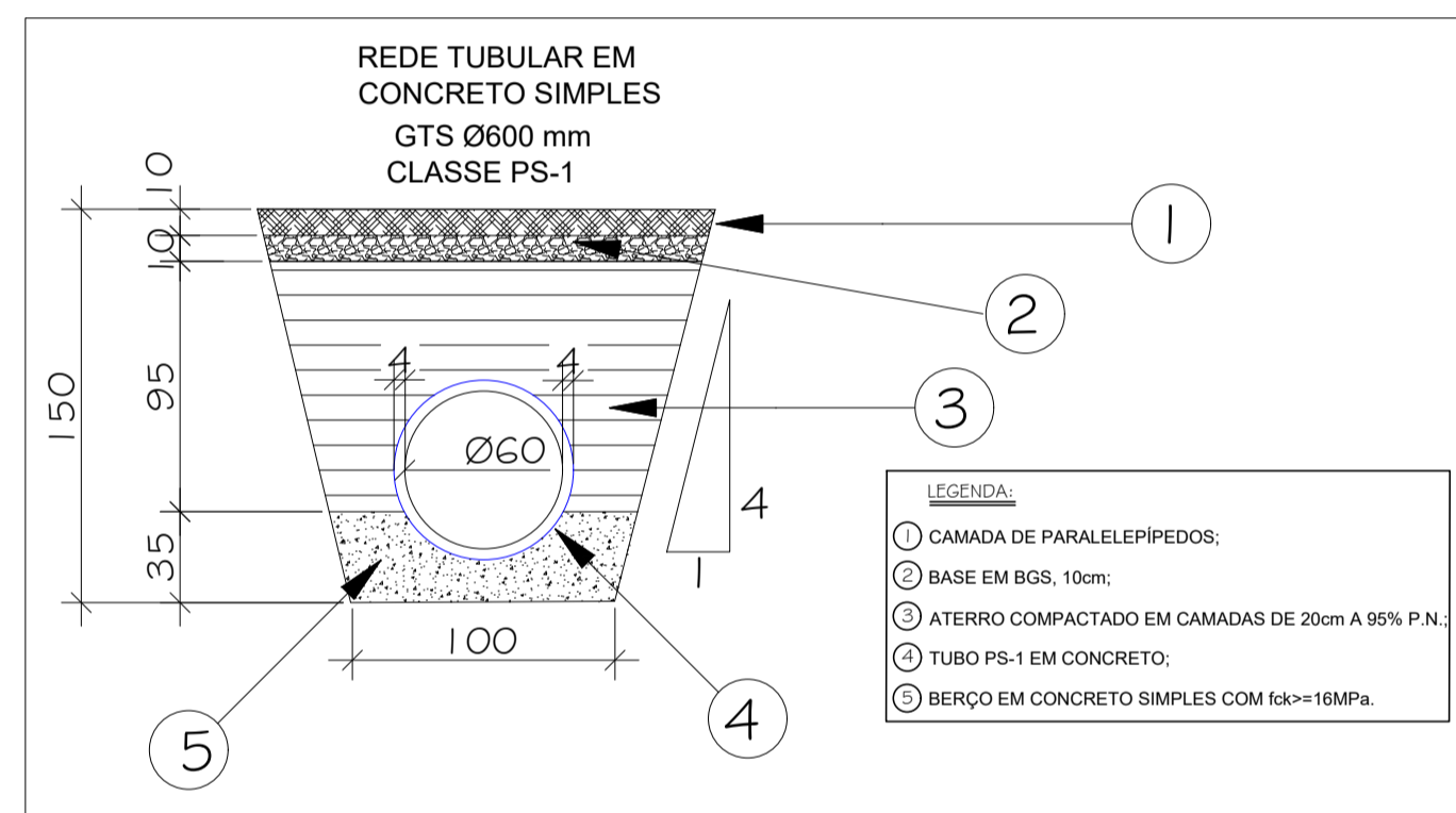
GTS 01 - #600mm - DETALHE ESCAVAÇÃO E BERÇO DE CONCRETO MAGRO SEM ESCALA
