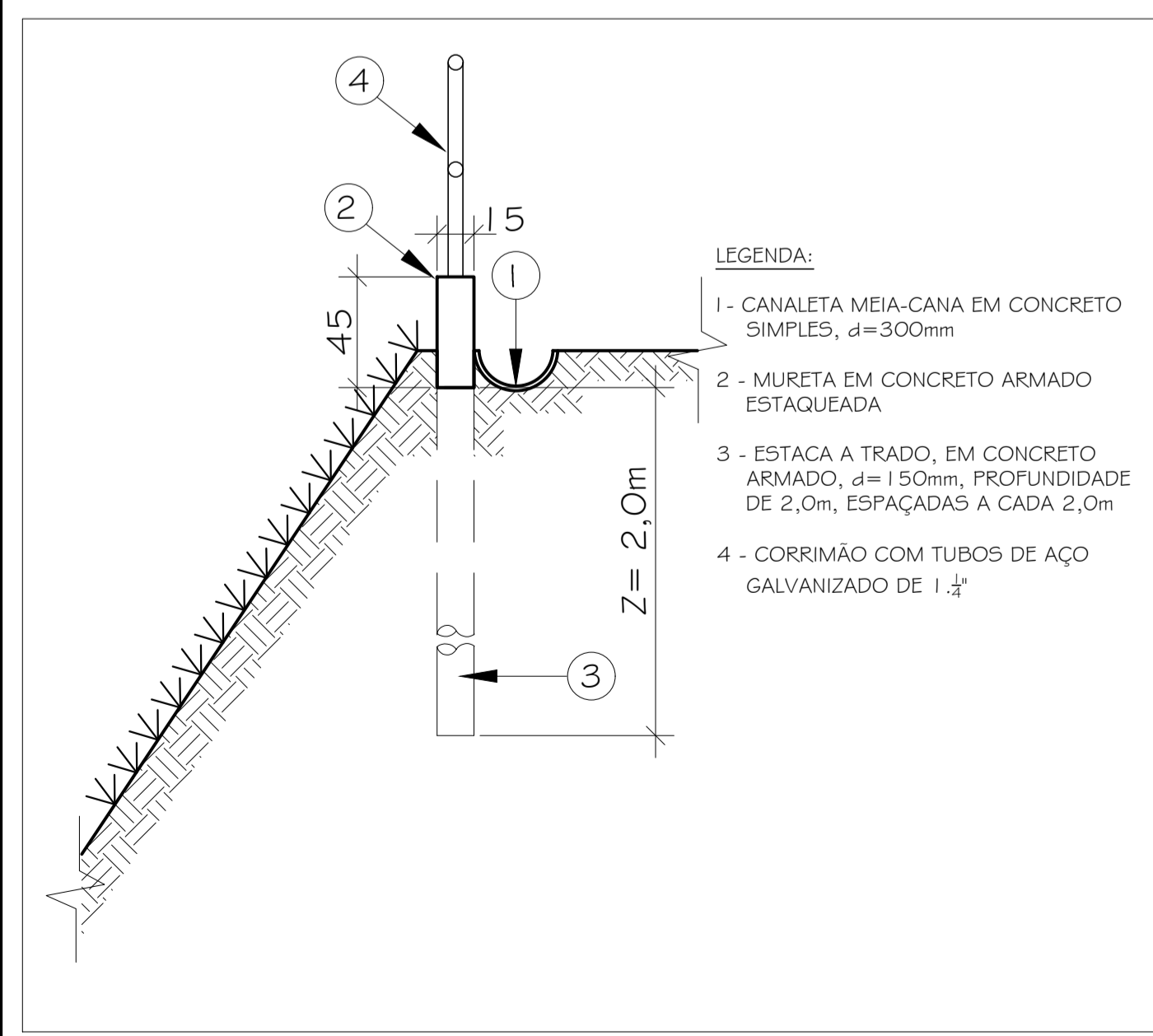
MEIO FIO COM ESTACA A TRADO - DETALHE TIPO SEM ESCALA
