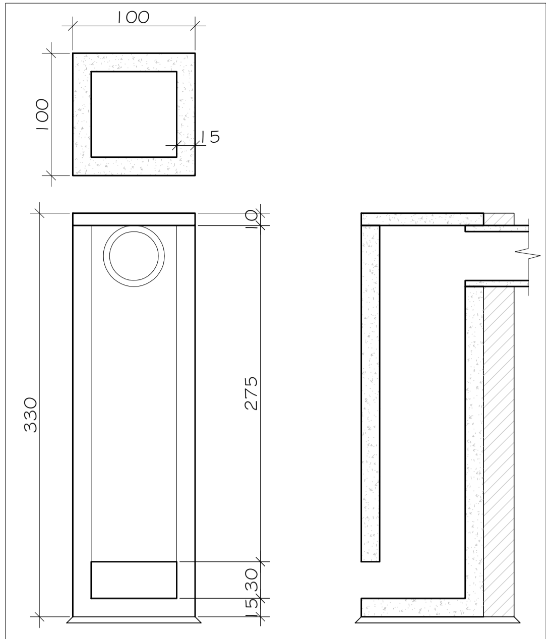
CONDUTO VERTICAL - h=3,30m - DETALHE TIPO SEM ESCALA
