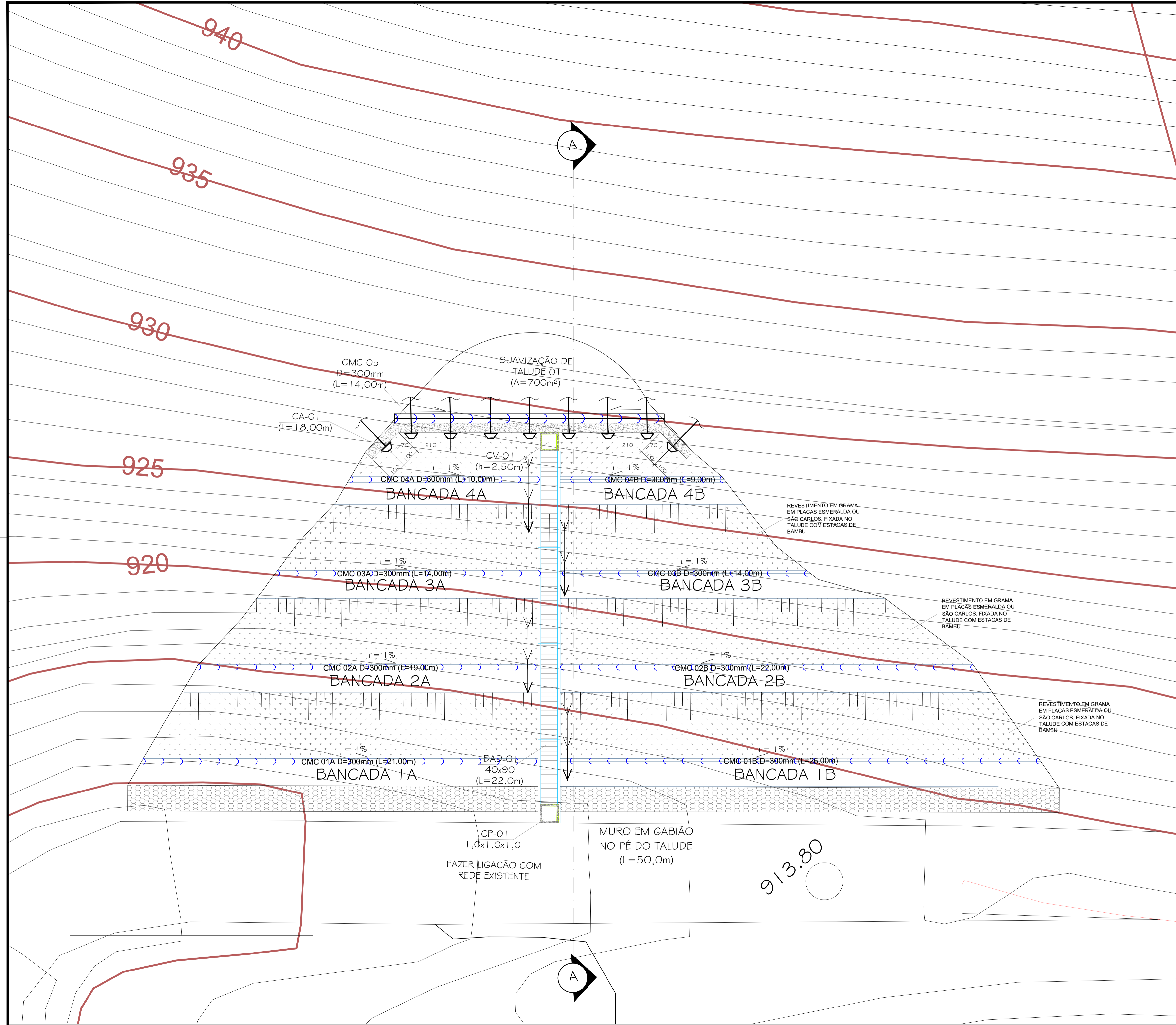
1 ARRANJO GERAL DE INTERVENÇÕES ESCALA 1/100
