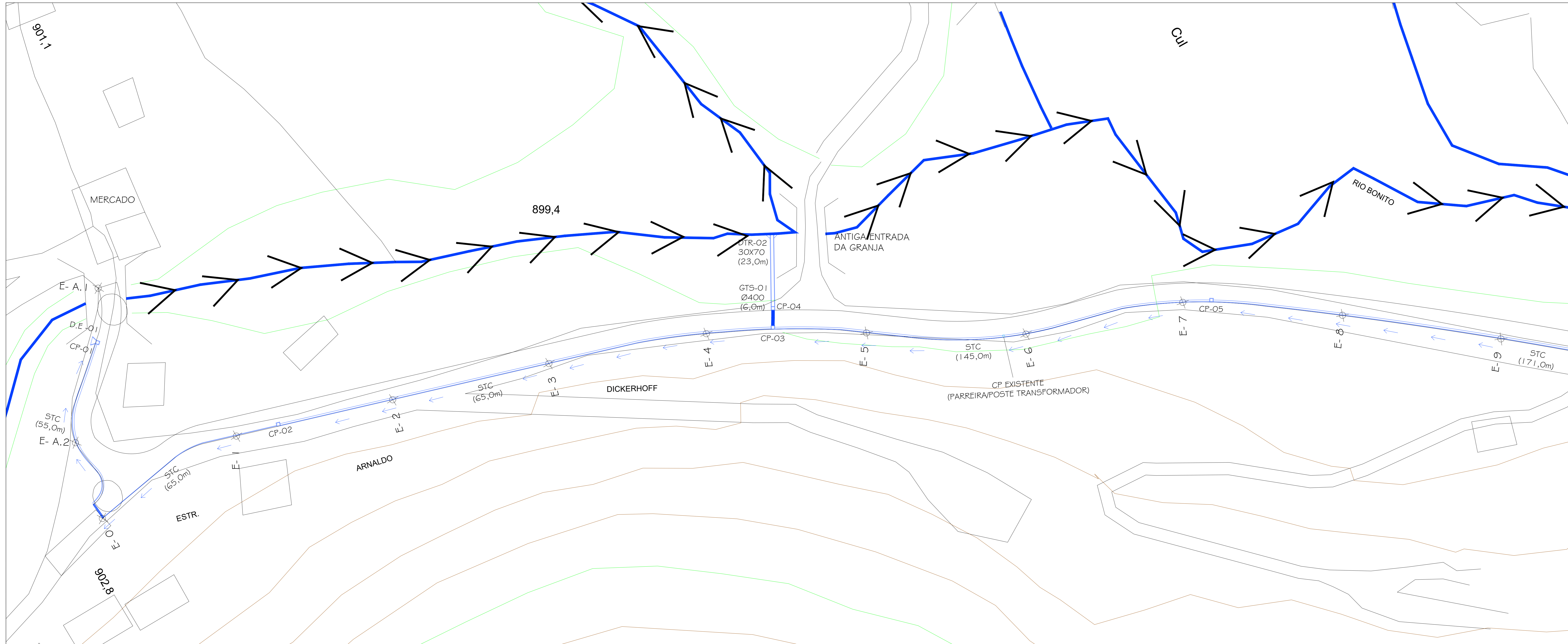
1 PLANTA DE DRENAGEM - TRECHO 01 - E0-E9 ESCALA 1/500
