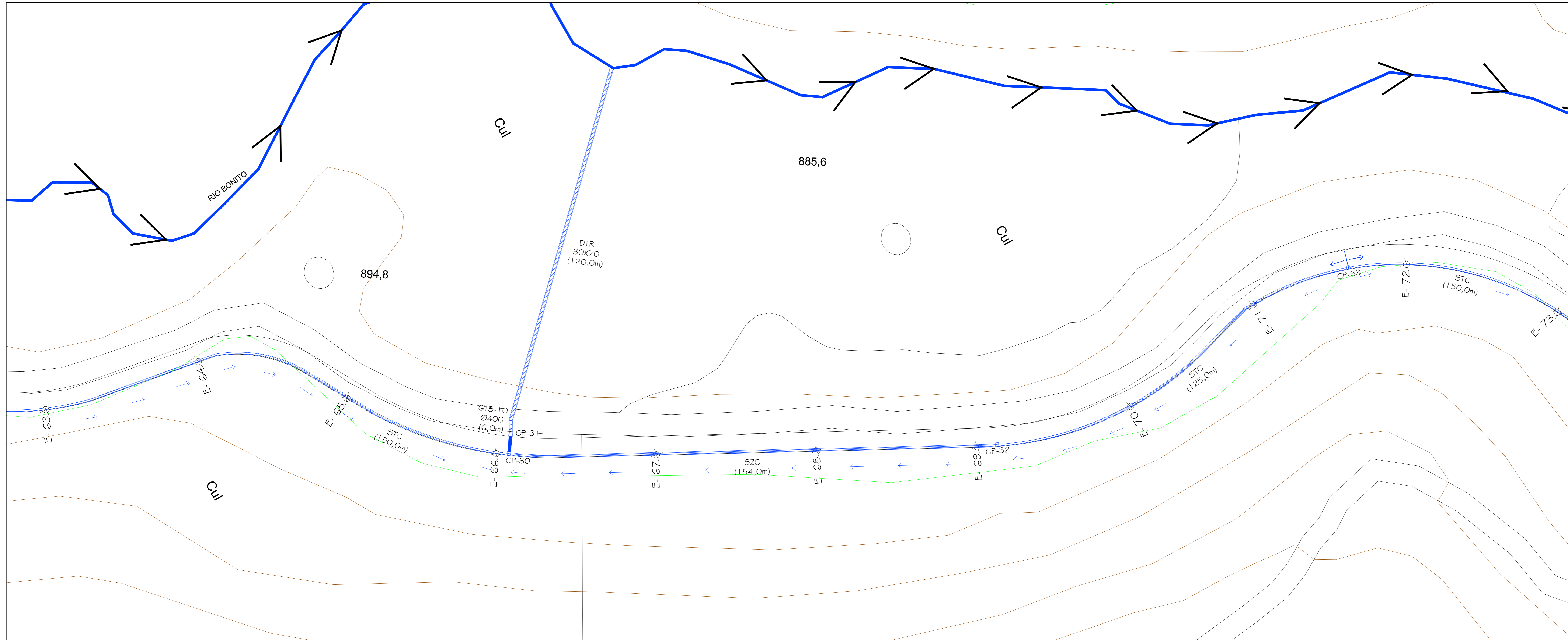
1 PLANTA DE DRENAGEM - TRECHO 07 - E63-E73
