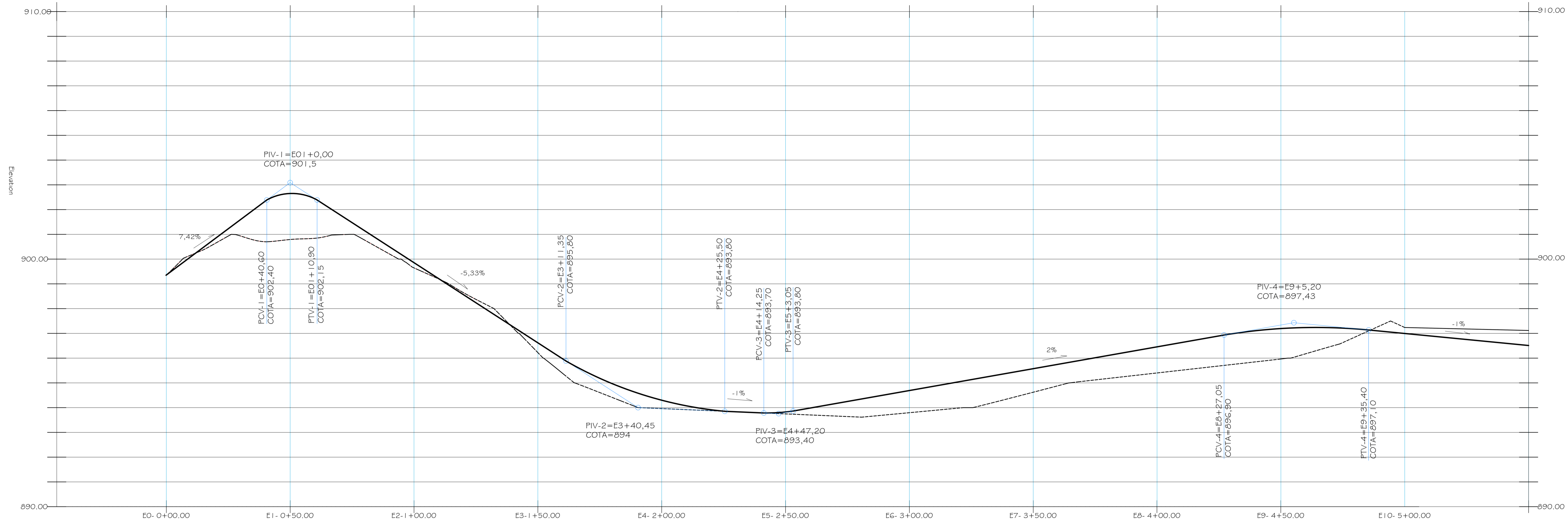
1 PERFIL - TRECHO 01 ESCALA HORIZONTAL: 1/750 - ESCALA VERTICAL: 1/75
