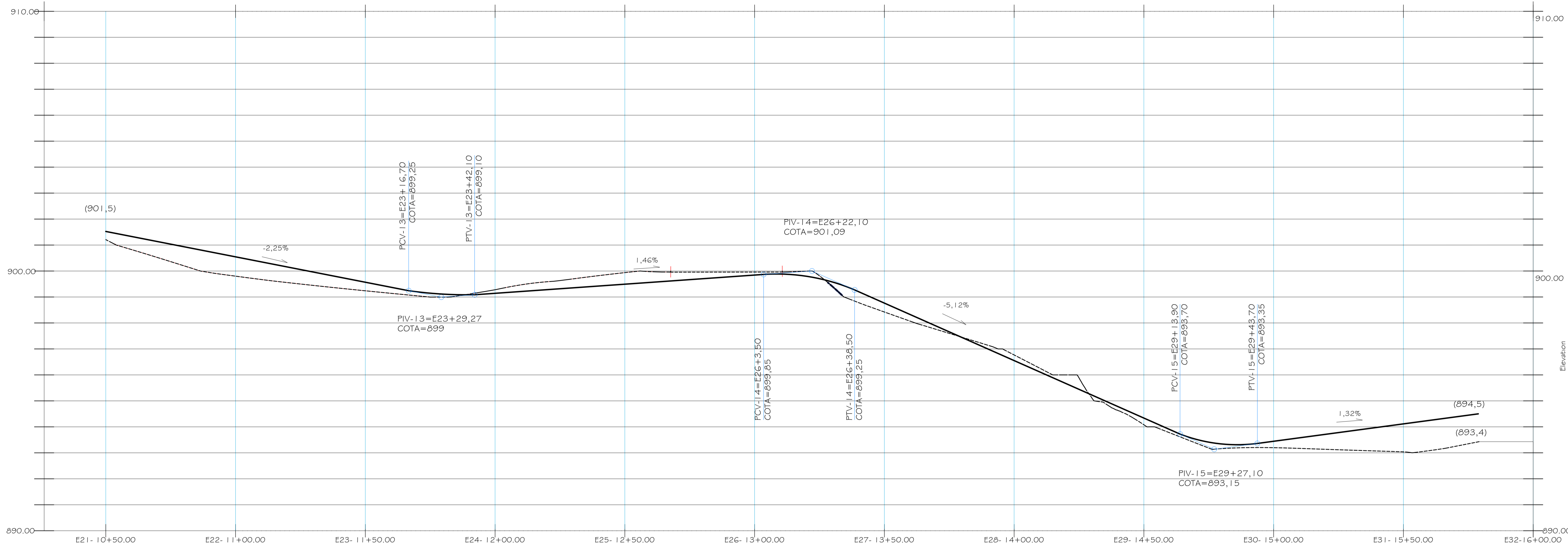
1 PERFIL - TRECHO 03 ESCALA HORIZONTAL: 1/750 - ESCALA VERTICAL: 1/75
