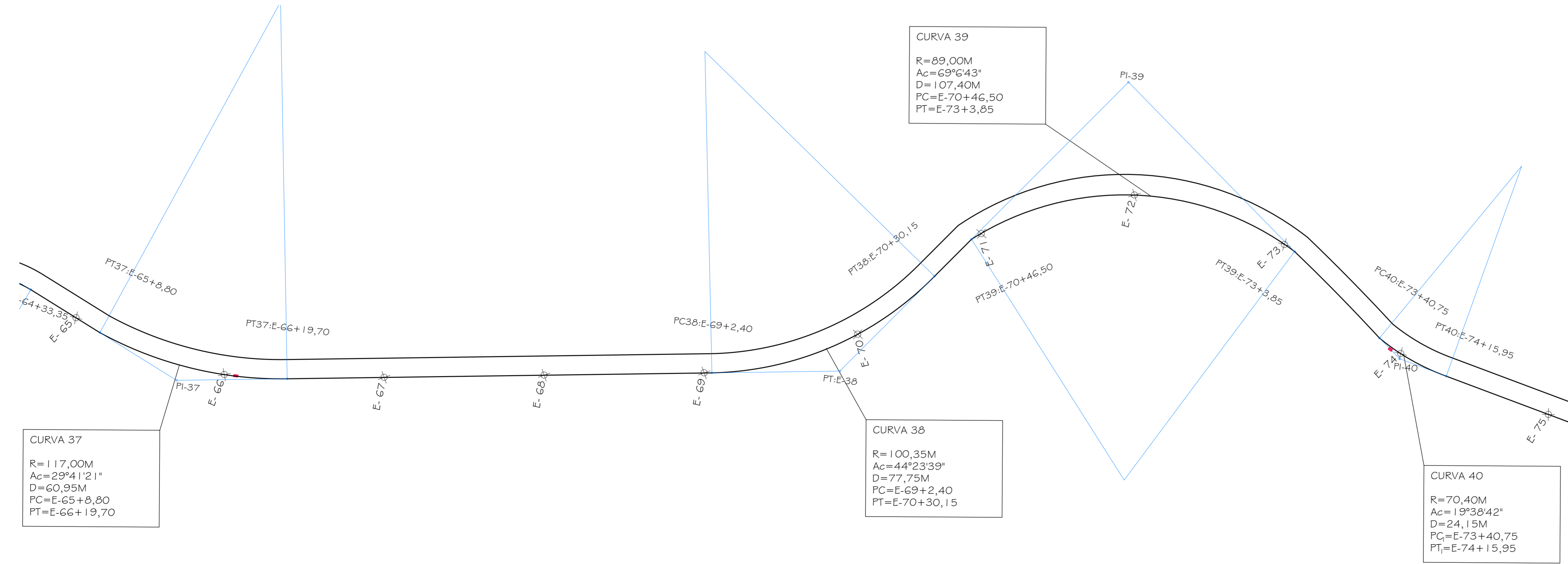
2 ESTRADA ARNALDO DIECKENHOFF - TRECHO 07 - E65-E76 ESCALA 1/750
