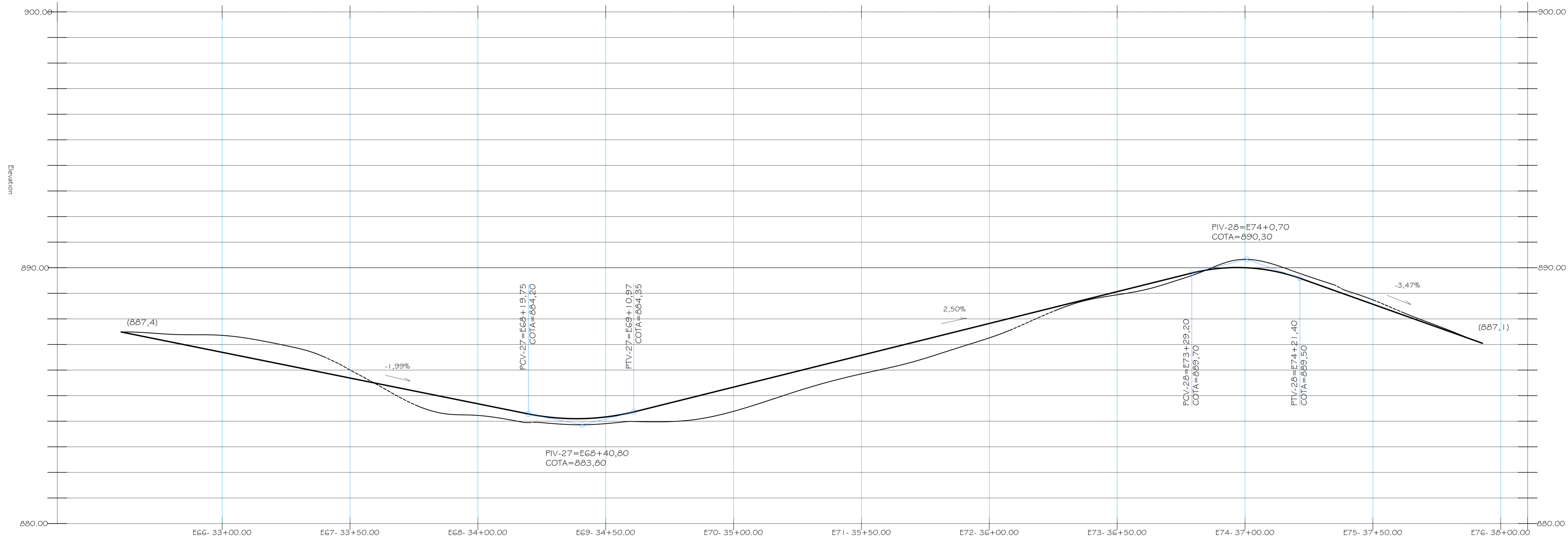
1 PERFIL - TRECHO 07 ESCALA HORIZONTAL: 1/750 - ESCALA VERTICAL: 1/75
