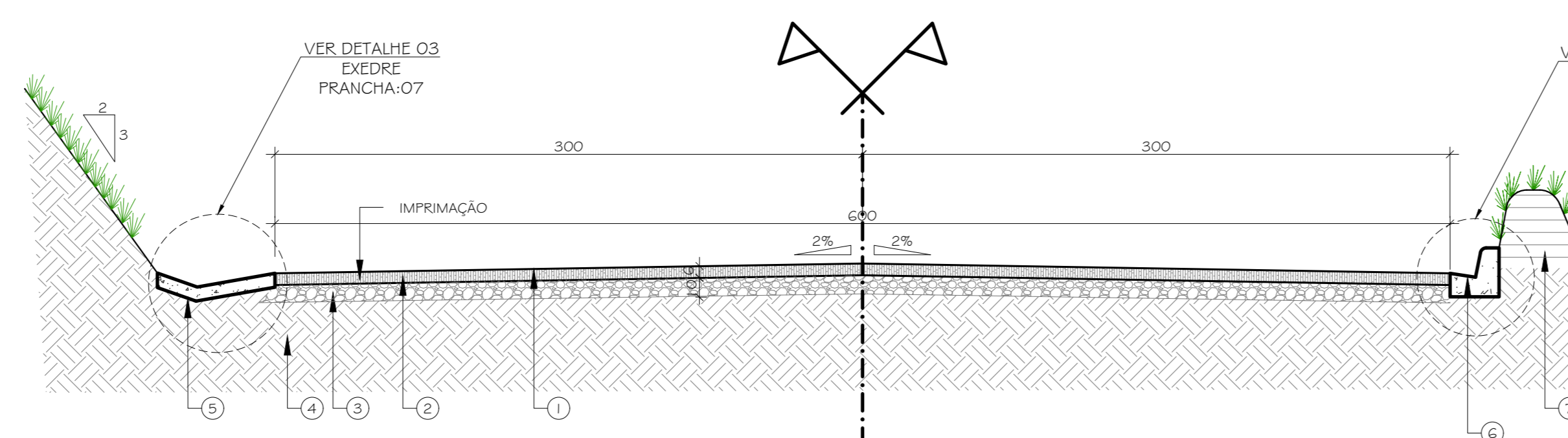
3 SEÇÃO TRANSVERSAL - E63+14-E66+4 / E69+7-E71+32 ESCALA 1/25
