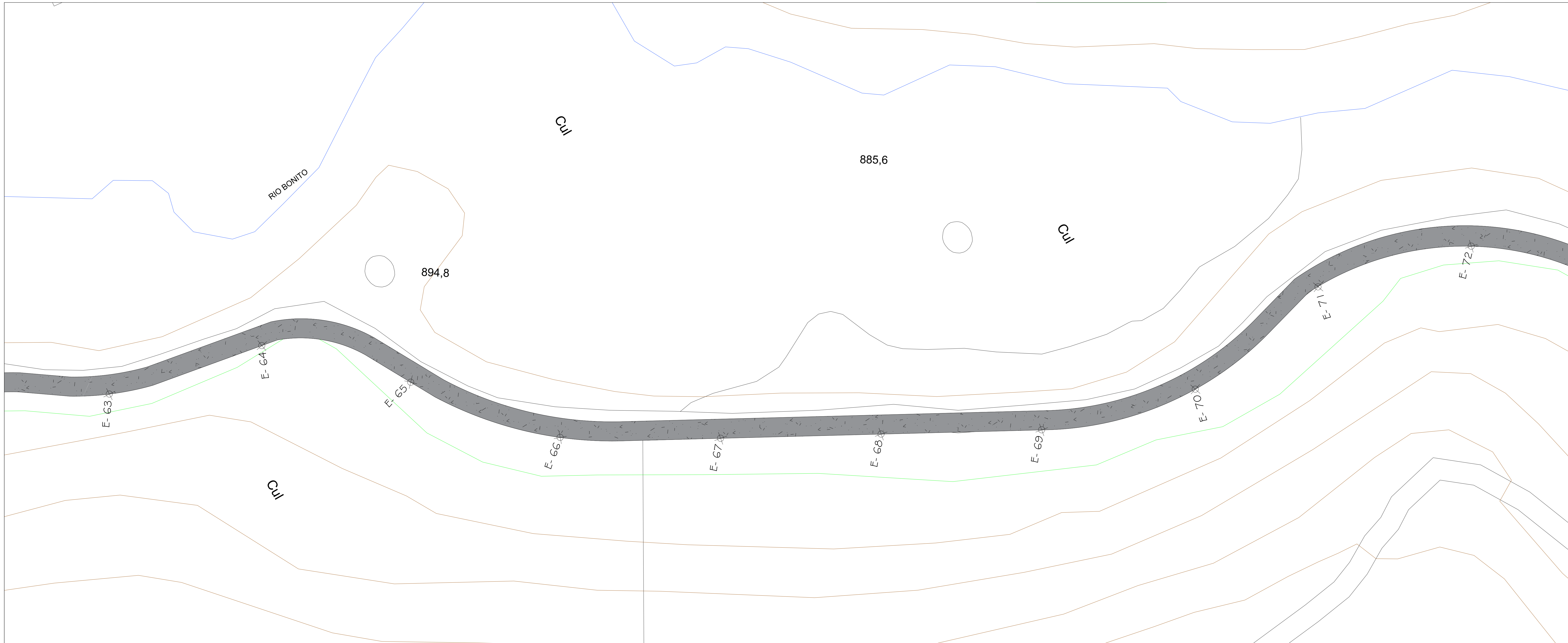
1 PLANTA DE PAVIMENTAÇÃO - TRECHO 07 - E63-E72 ESCALA 1/500
