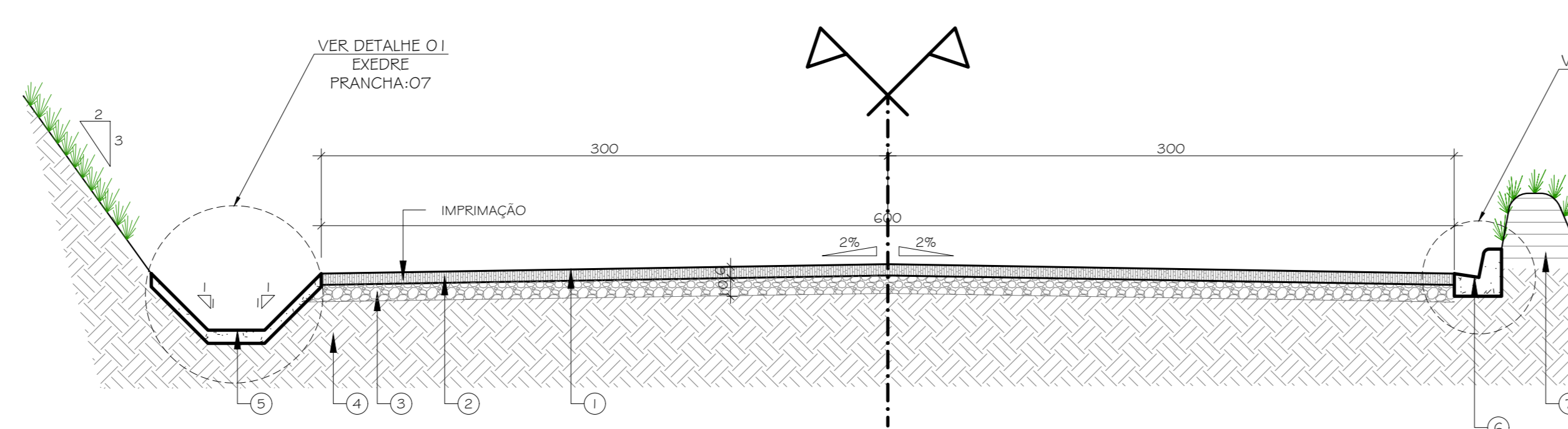
2 SEÇÃO TRANSVERSAL - E66+4-E69+7 ESCALA 1/25
