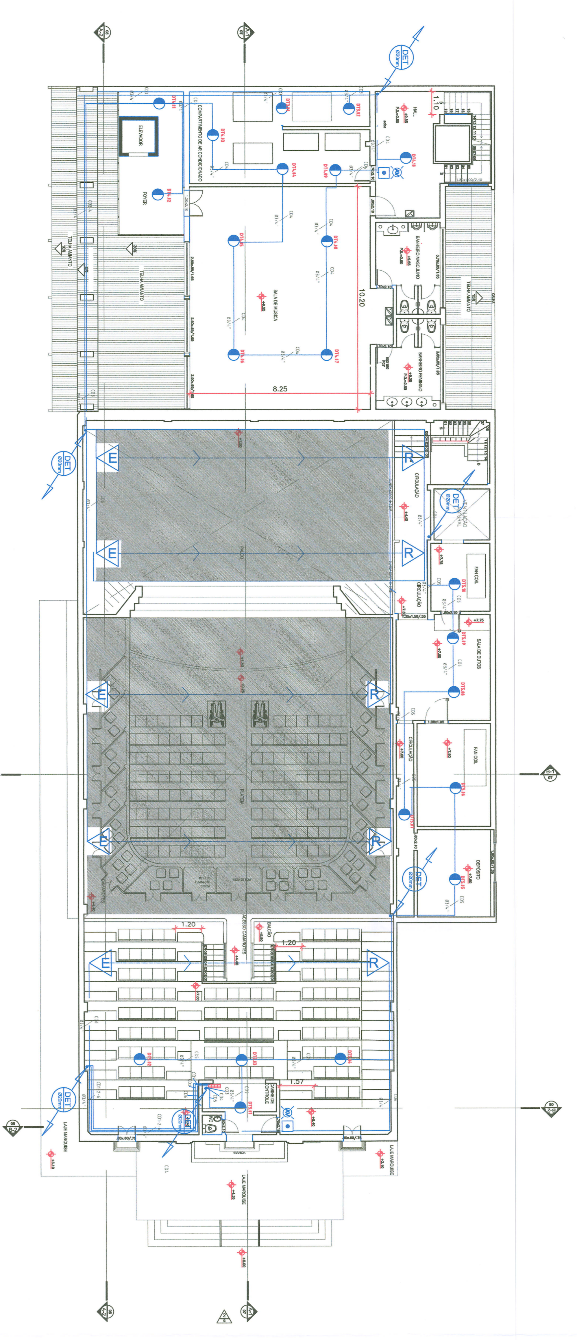
1 PLANTA BAIXA 2º PAVIMENTO Esc.: 1/100
