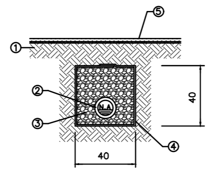
SEÇÃO TIPO DA VALA DE TUBULAÇÃO PEAD SEM ESCALA
