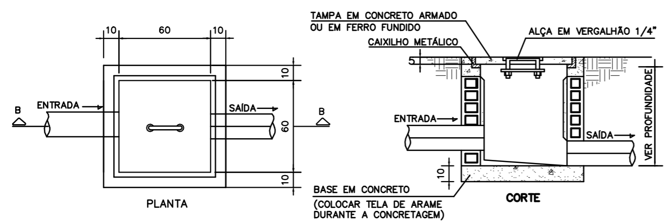
CAIXA DE AREIA PARA ÁGUA PLUVIAL SEM ESCALA
