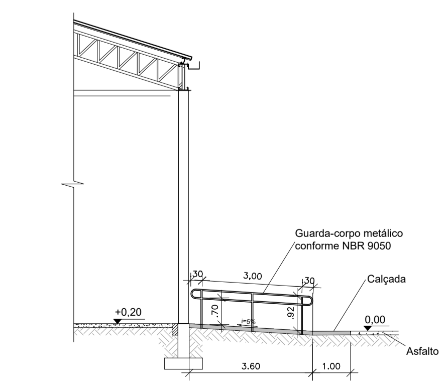
3 DET 01 - RAMP/GUARDA CORPO ESCALA 1/100
