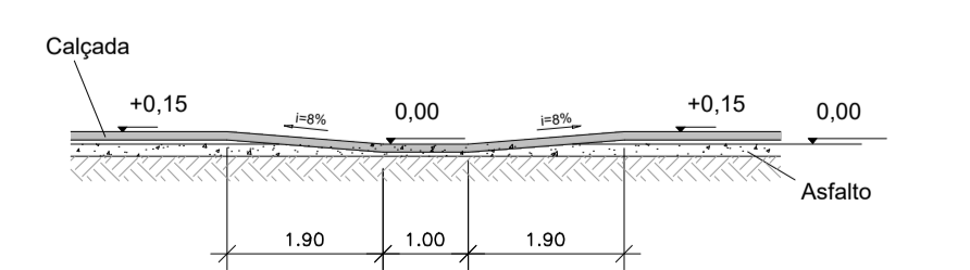
4 DET 02 - RAMP/ CALÇADA ESCALA 1/100
