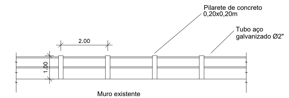
5 DET 03 - GUARDA-CORPO ESCALA 1/100
